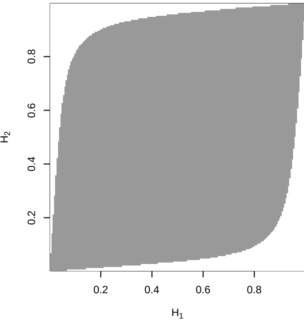
\rho = 0.5
