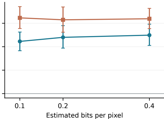
YUV 6:1:1 PSNR
