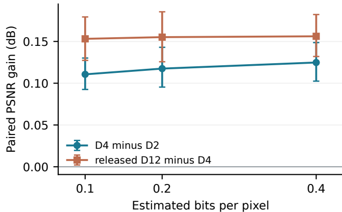
RGB PSNR
