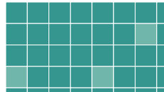
Bayer dither
