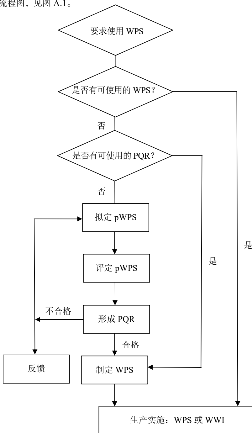
图 A.1 焊接工艺规程流程图
