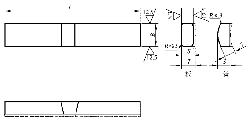
a) 板状和管状试件的面弯试样
