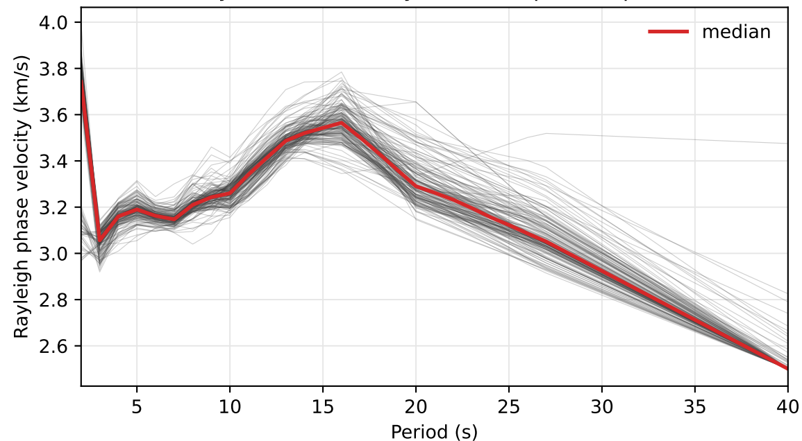
Bayan Obo subarray MASW dispersion picks
