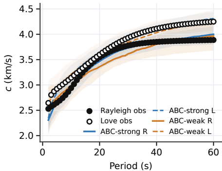
Reference posterior predictive
