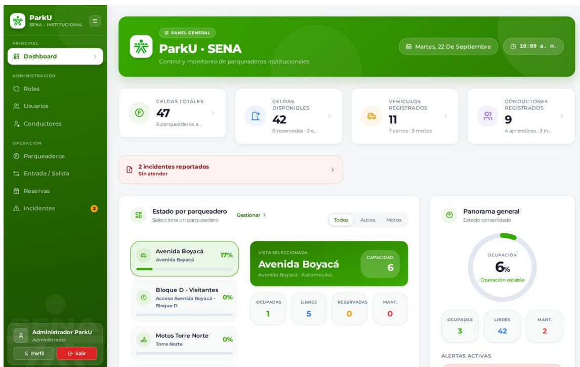
Figura 20. Estructura general de la aplicación (vista del Administrador)
