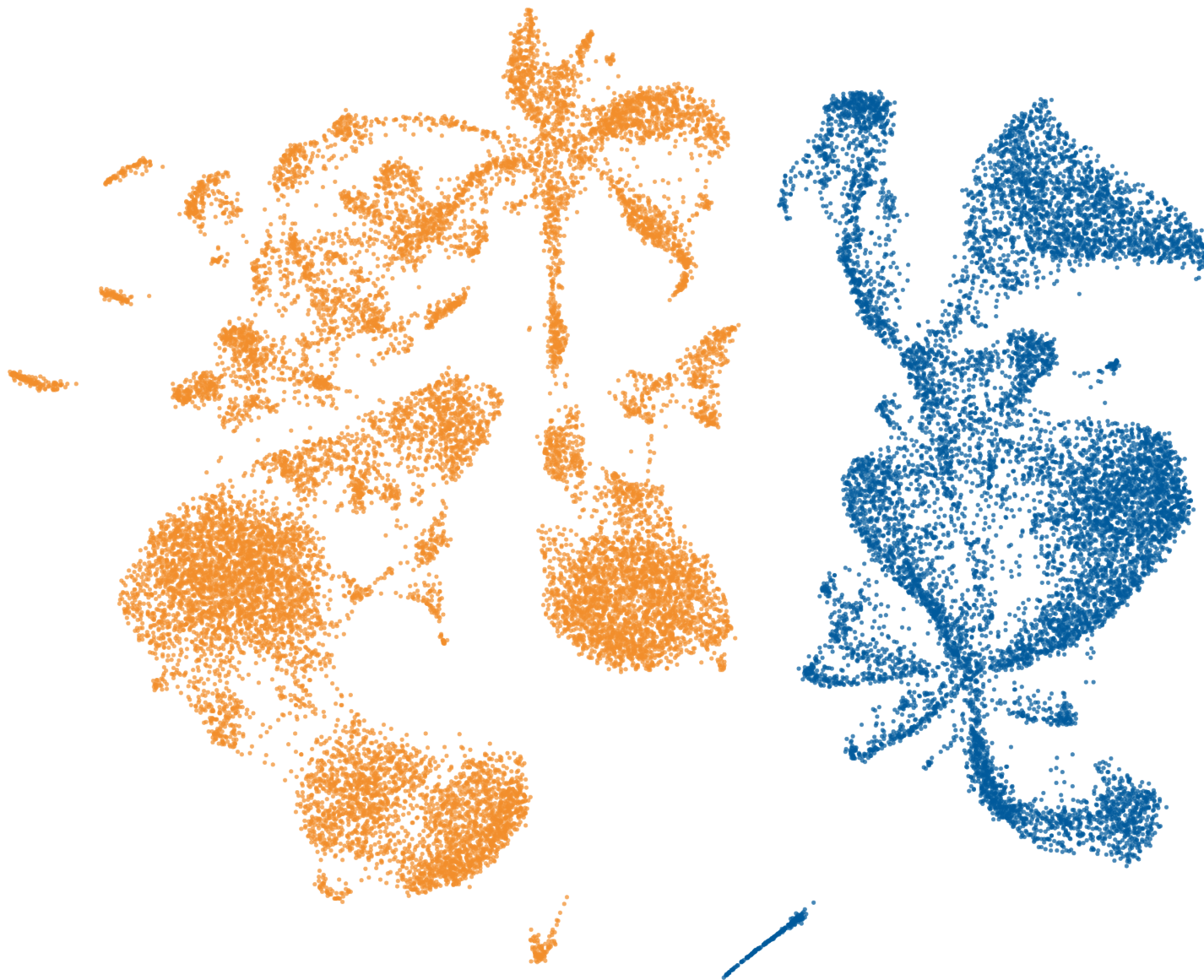
PCA — Species
