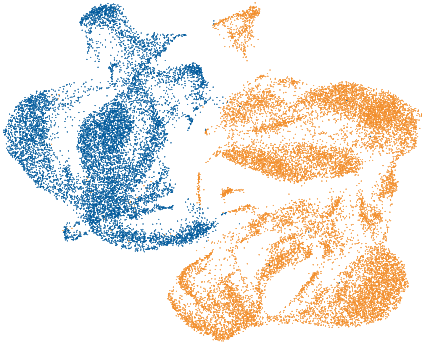
TranscriptFormer — Species
