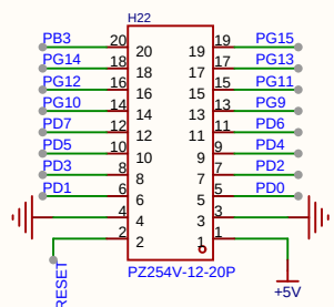
核心板接口
