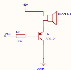
蜂鸣器
