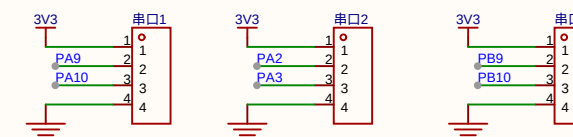
串口1
