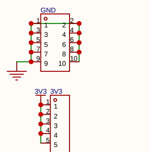
电源接口
