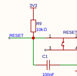
复位按键
