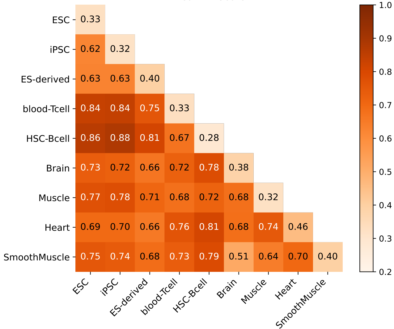
Mean F1 Score
