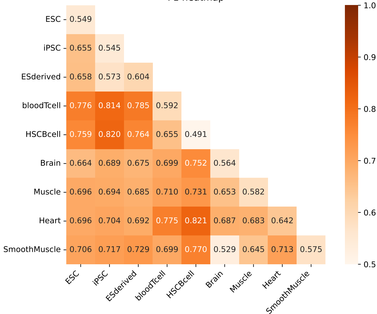
F1 heatmap
