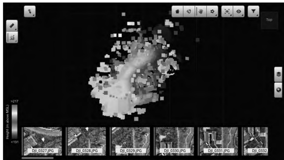
图1 ContextCapture高差图
