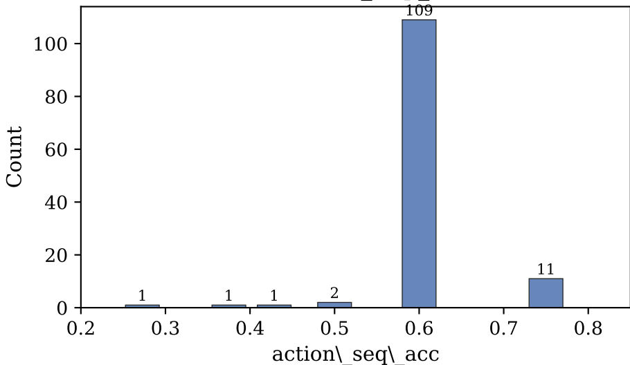
Qwen-3B: action\_seq\_acc (N=8)
