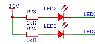
预留LED指示灯
