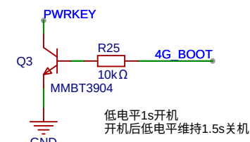
LTE开关机控制
