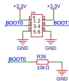
STM32启动控制
