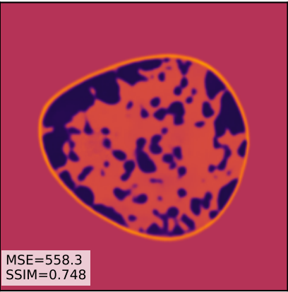
InversionNet
