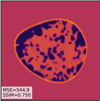
PGCR
