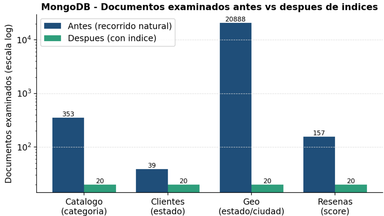
Figura 5. MongoDB: documentos examinados antes vs despues de indices.
