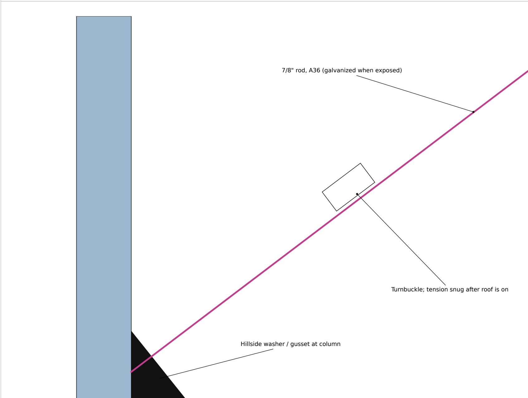
7 ROD X-BRACE END SCALE: NTS
