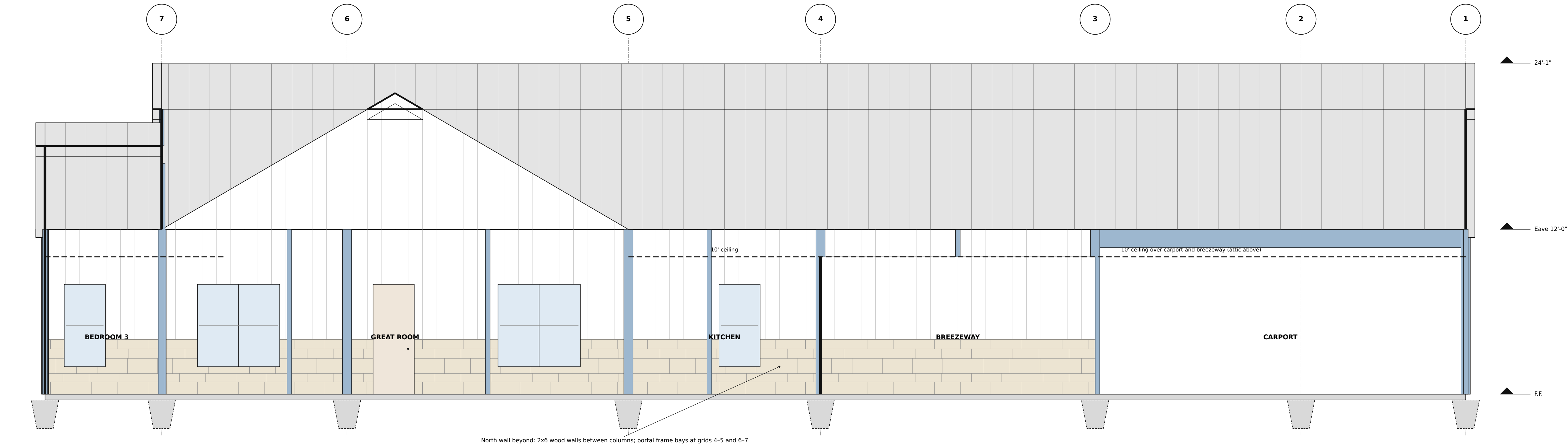
2 SECTION 2 — LONGITUDINAL SCALE: 1/4" = 1'-0"
