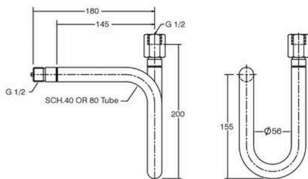
"U" Type Siphon DIN
