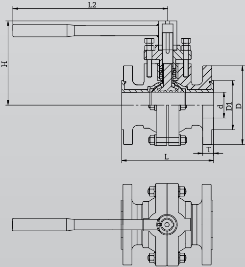
DIMENSIONS
