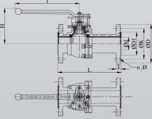
DIMENSIONS
