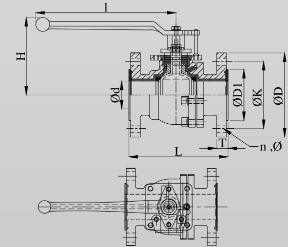
DIMENSIONS
