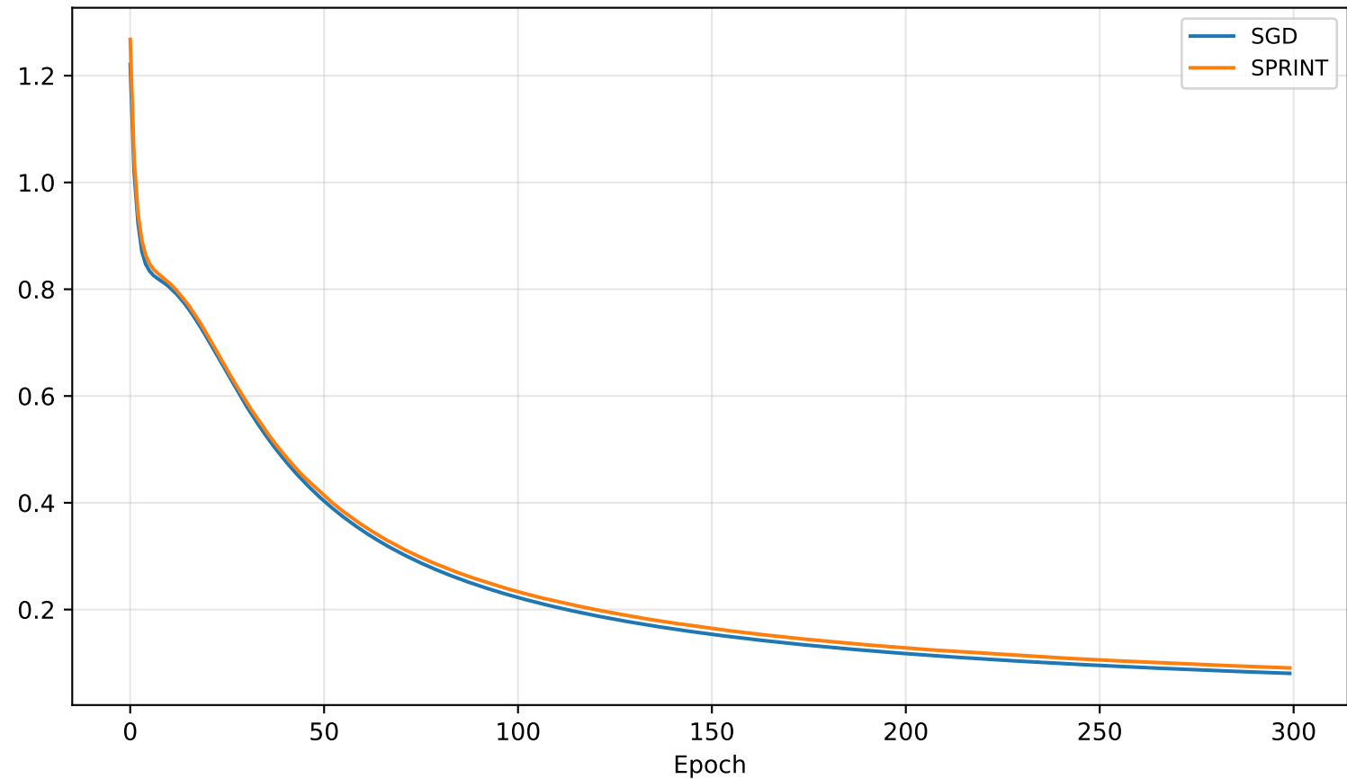
Gradients Norm
