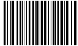
Code 128
