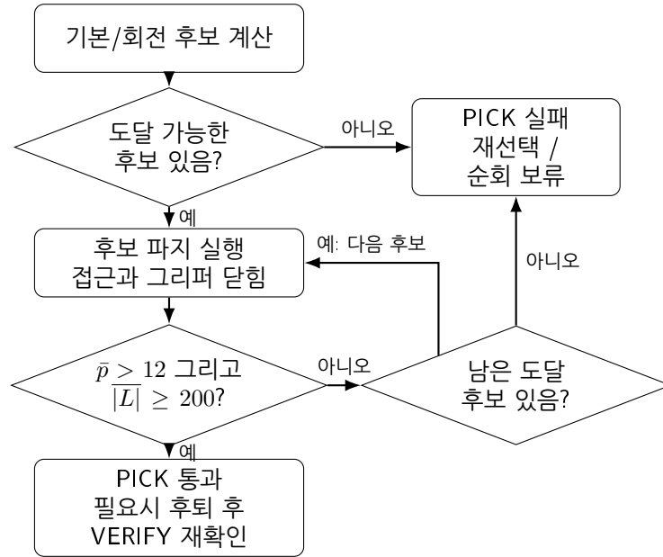
그림 3.5: PICK 내부의 후보 시도와 센서 판정. \bar{p} 와 |\overline{L}| 은 위치와 절대 부하의 표본 평균이며, 표시한 임계값은 현재 설정이다. 개별 동작 시간 초과는 PICK 실패로 처리하며, 외부 180초 종료와 구분한다.
