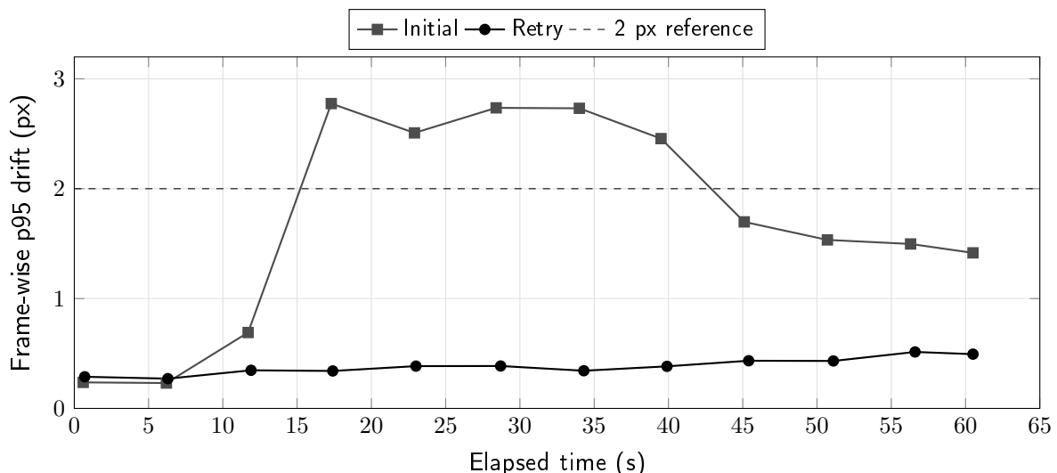
그림 4.4: 초기 검사와 재검사의 표본별 드리프트 p95. 점선은 2 pixel 기준값이다.
