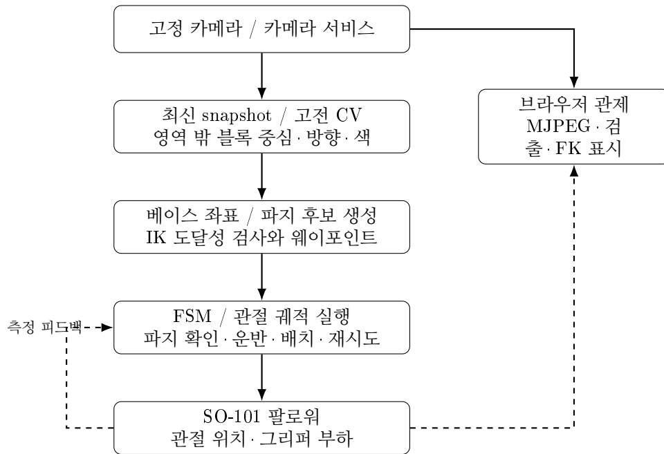
그림 3.1: 기본 CV+IK 제어 경로와 관제 구성. 실선은 주 입력 · 실행 경로, 점선은 측정 상태의 전달이다. 추가 관측 기능은 절 3.6.2에서 설명한다.
