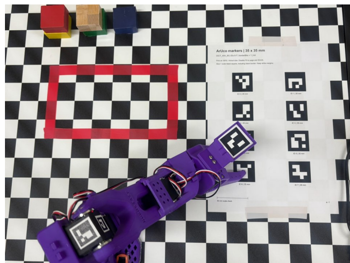
그림 3.7: 그리퍼에 부착한 ArUco 마커(35×35 mm)와 마커 시트, 체커보드, 대상 블록. 상단·하단 두 지점에 마커를 부착하여 그리퍼 자세를 함께 추정할 수 있도록 하였다.
