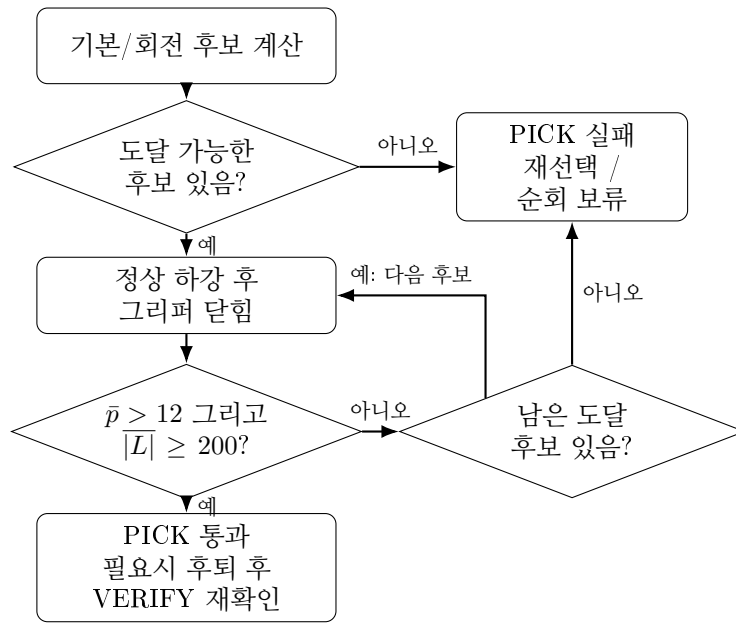
그림 3.5: PICK의 후보 선택과 정상 하강 후 센서 판정. 하강이 막힌 후보는 그리퍼를 닫지 않고 후퇴하여 다음 후보로 넘어간다. \bar{p} 와 |\bar{L}| 은 위치와 절대 부하의 표본 평균이며, 표시한 임계값은 평가에 사용한 설정이다. 개별 동작 시간 초과는 PICK 실패로 처리하며, 외부 180 초 종료와 구분한다.
