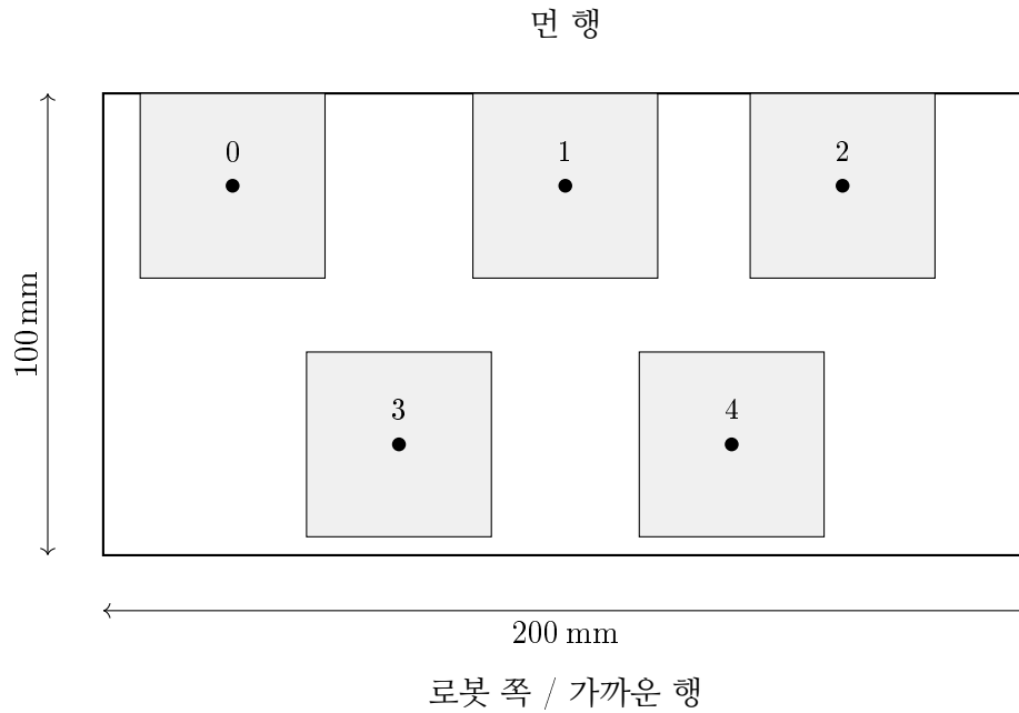
그림 3.8: 200 × 100 mm 지정 영역의 3+2 슬롯 설계. 사각형은 40 mm 블록의 명목 크기, 숫자는 슬롯 번호이다.
