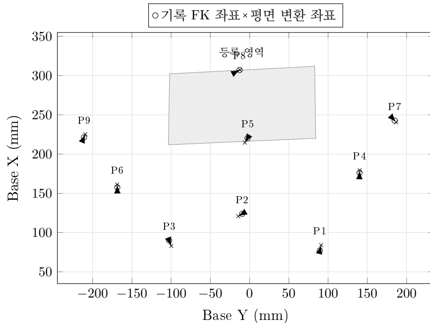
그림 4.1: 최종 대응점의 FK 좌표와 평면 변환 좌표. 화살표는 적합 잔차를 실제 축척으로 표시하며, 음영은 등록된 지정 영역이다.
