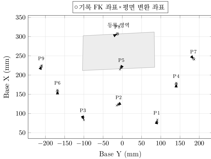
그림 4.3: 최신 대응점의 FK 좌표와 평면 변환 좌표. 화살표는 두 좌표의 차이를 실제 축척으로 표시한다. 음영은 같은 프로필의 등록 영역이며, 이 그림은 물리적인 텍 위치의 독립 측정 결과가 아니다.
