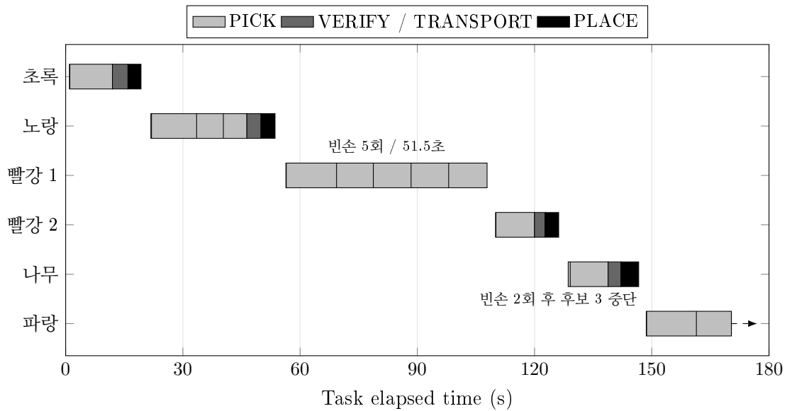
그림 4.6: 9월 8일 진단 시험의 상태별 실행 시간. PICK 내부의 세로선은 후보 시작이며, 빨강 1과 2는 재선택 전후이다. 빈 구간에는 SELECT가 포함된다. 파랑의 점선은 마지막 후보 시작 뒤 중단을 뜻하며 정확한 중단 시각이나 소요시간을 나타내지 않는다.
