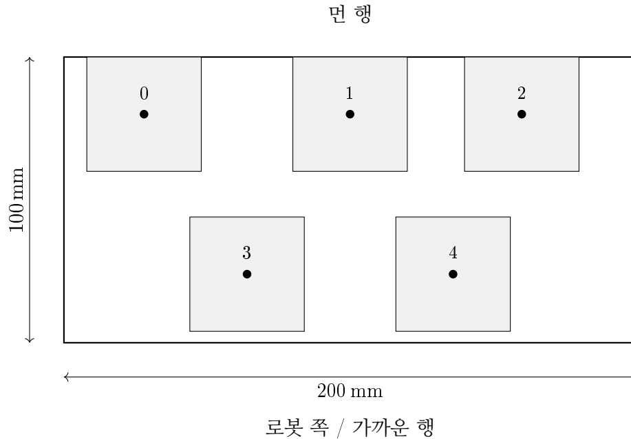
그림 3.5: 200 × 100 mm 지정 영역의 3+2 슬롯 설계. 사각형은 40 mm 블록의 명목 크기, 숫자는 슬롯 번호이다.
