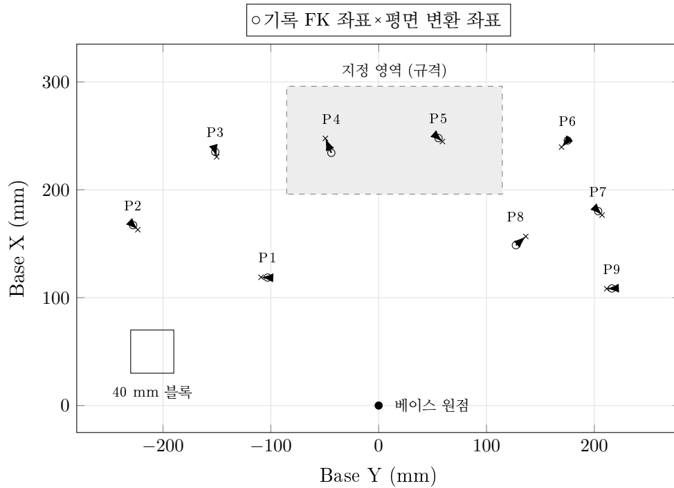
그림 4.2: 작업 평면의 대응점과 적합 잔차 방향. 음영은 200 \times 100 mm 지정 영역의 개략도이다. 원에서 십자로 향하는 화살표는 기록 FK 좌표에서 평면 변환 좌표까지의 차이이며 실제 크기로 표시하였다. P1은 재수집점이다. 실제 텍 오차나 LOO 벡터를 측정한 그림은 아니다.
