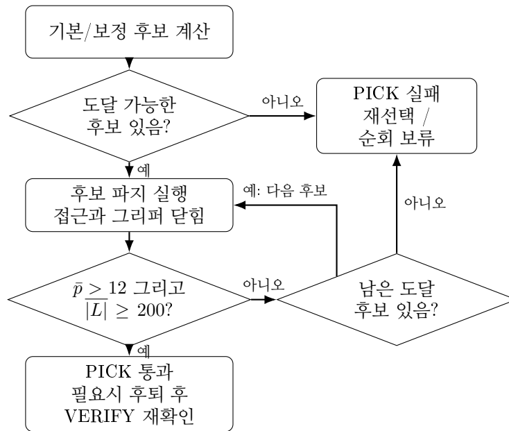
그림 3.4: PICK 내부의 후보 시도와 센서 판정. \bar{p} 와 |L| 은 위치와 절대 부하의 표본 평균이며, 표시한 임계값은 현재 설정이다. 동작 시간 초과도 PICK 실패로 처리한다.
