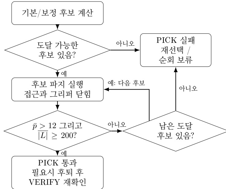
그림 3.3: PICK 내부의 후보 시도와 센서 판정. \bar{p} 와 |L| 은 위치와 절대 부하의 표본 평균이며, 표시한 임계값은 현재 설정이다. 동작 시간 초과도 PICK 실패로 처리한다.
