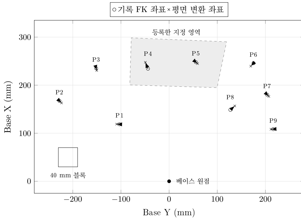
그림 4.2: 작업 평면의 대응점과 적합 잔차 방향. 원에서 십자로 향하는 화살표는 기록 FK 좌표에서 평면 변환 좌표까지의 차이이며 실제 크기로 표시하였다. P1은 재수집점이다. 실제 텍 오차나 LOO 벡터를 측정한 그림은 아니다.
