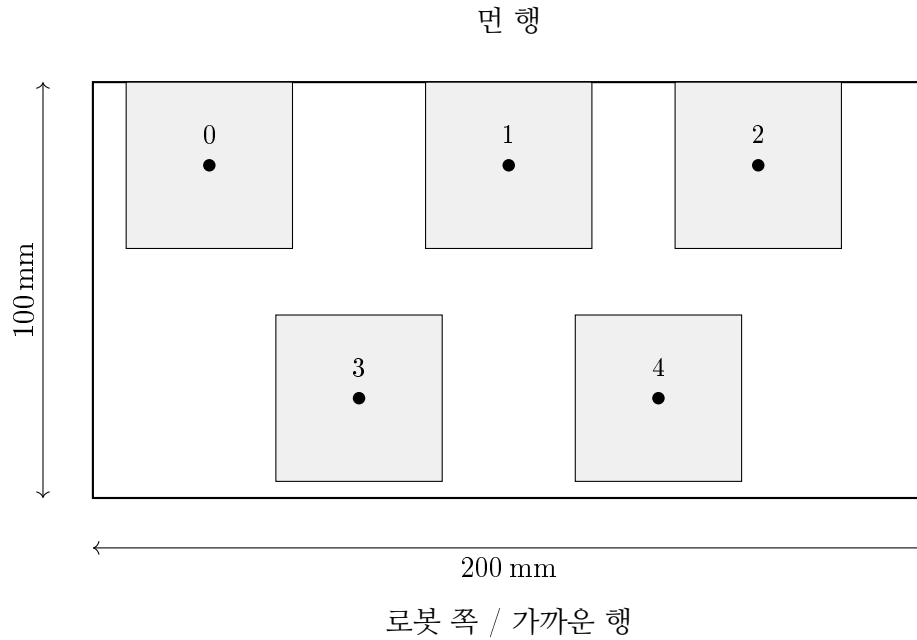
그림 3.4: 200 × 100 mm 지정 영역의 3+2 슬롯 설계. 사각형은 40 mm 블록의 명목 크기, 숫자는 슬롯 번호이다.
