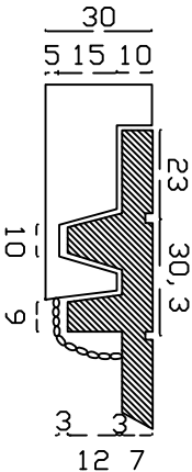
DETALLE B (tapa)
