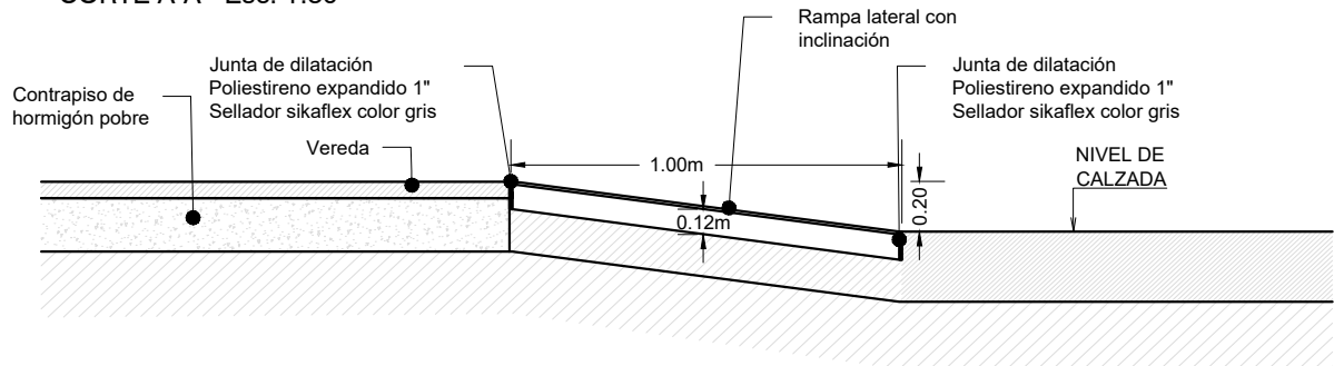
CORTE A-A - Esc. 1:30
