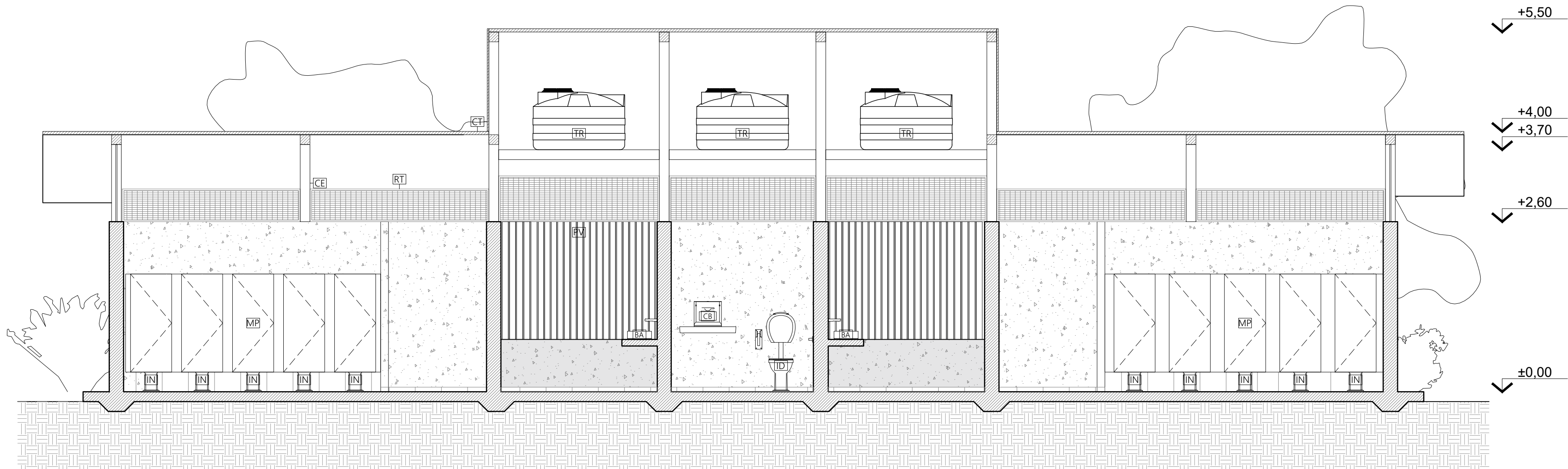
CORTE D-D ESC 1:50
