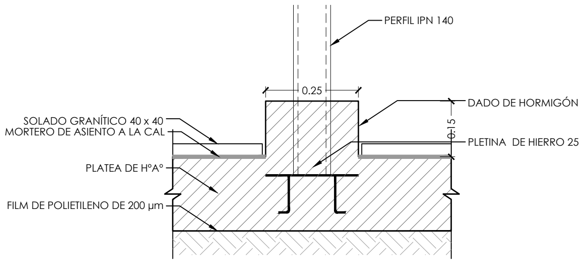
DETALLE FUNDACIÓN PÉRGOLA
