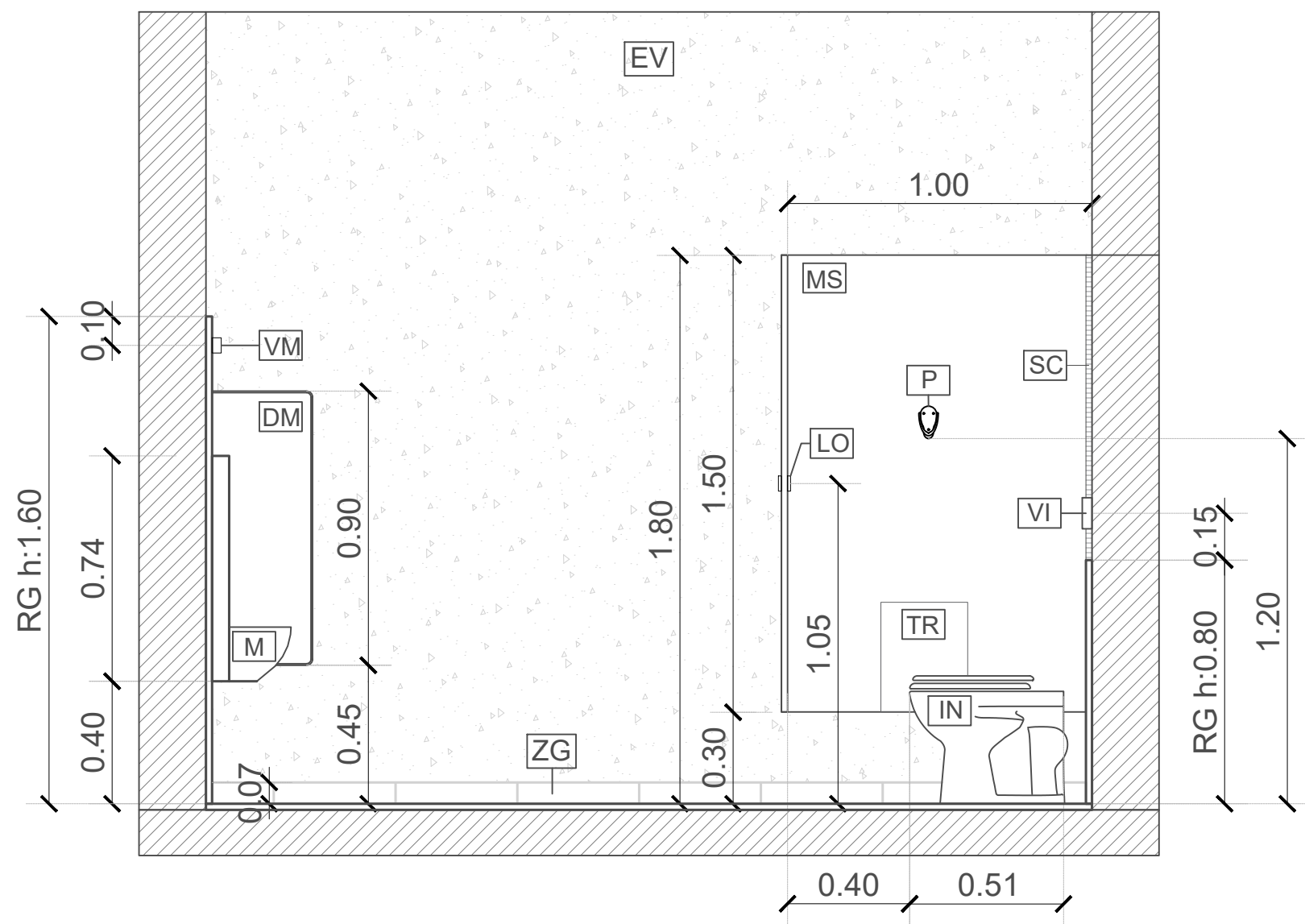
CORTE INODOROS BAÑO HOMBRES ESC 1:50
