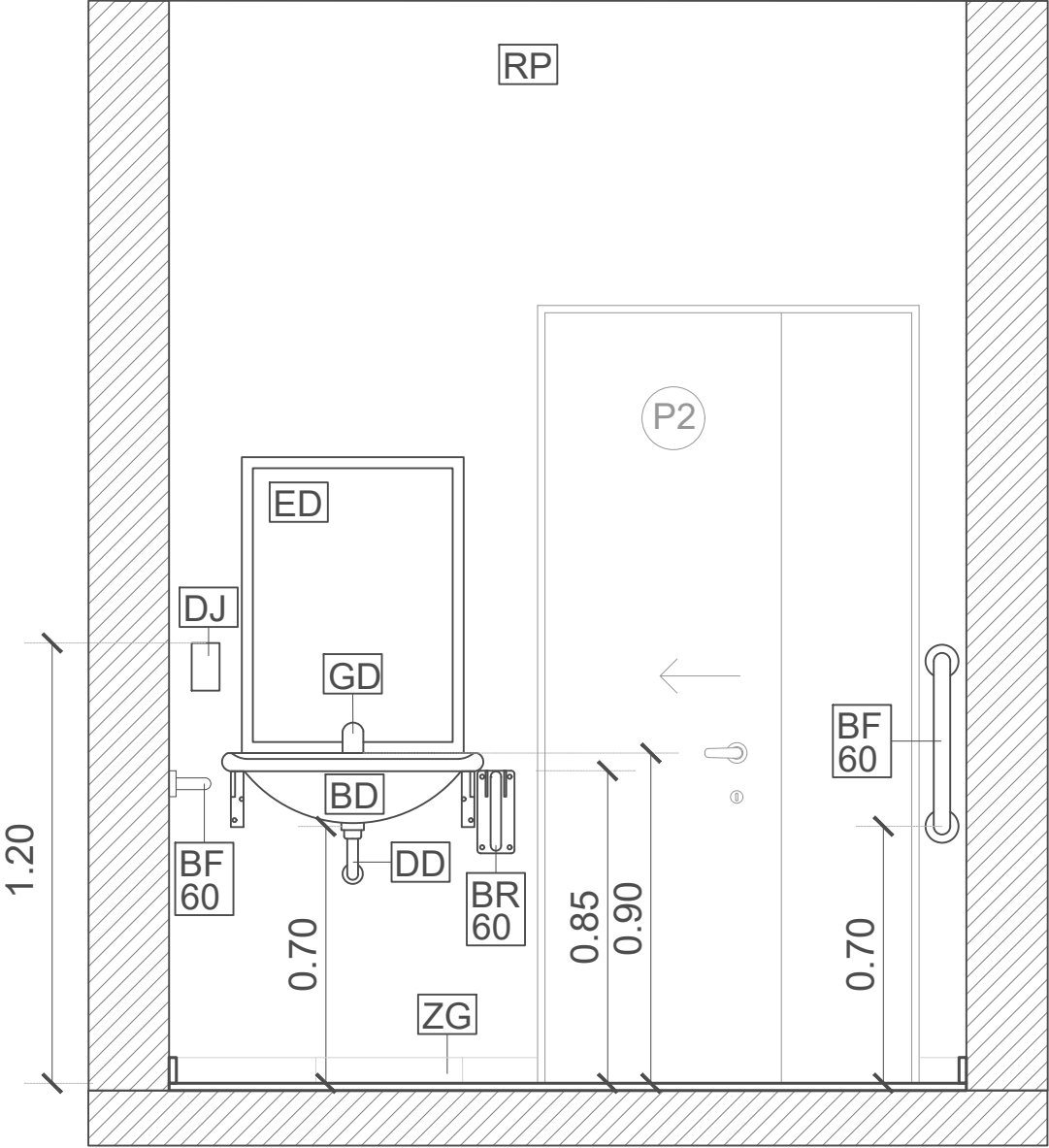
CORTE C - C ESC 1:50
