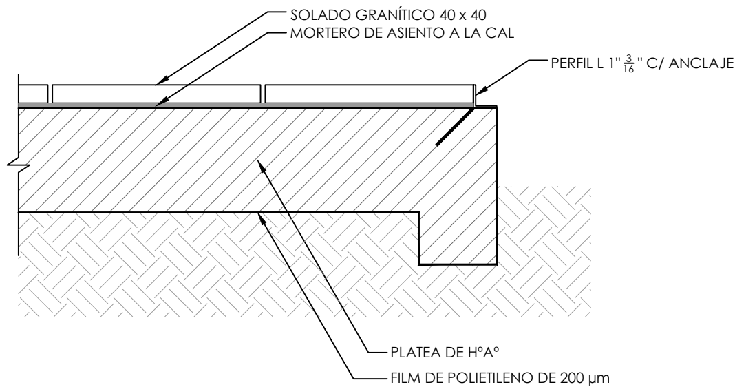
DETALLE PERFIL L DE TERMINACIÓN PLATEA DE FUNDACIÓN
