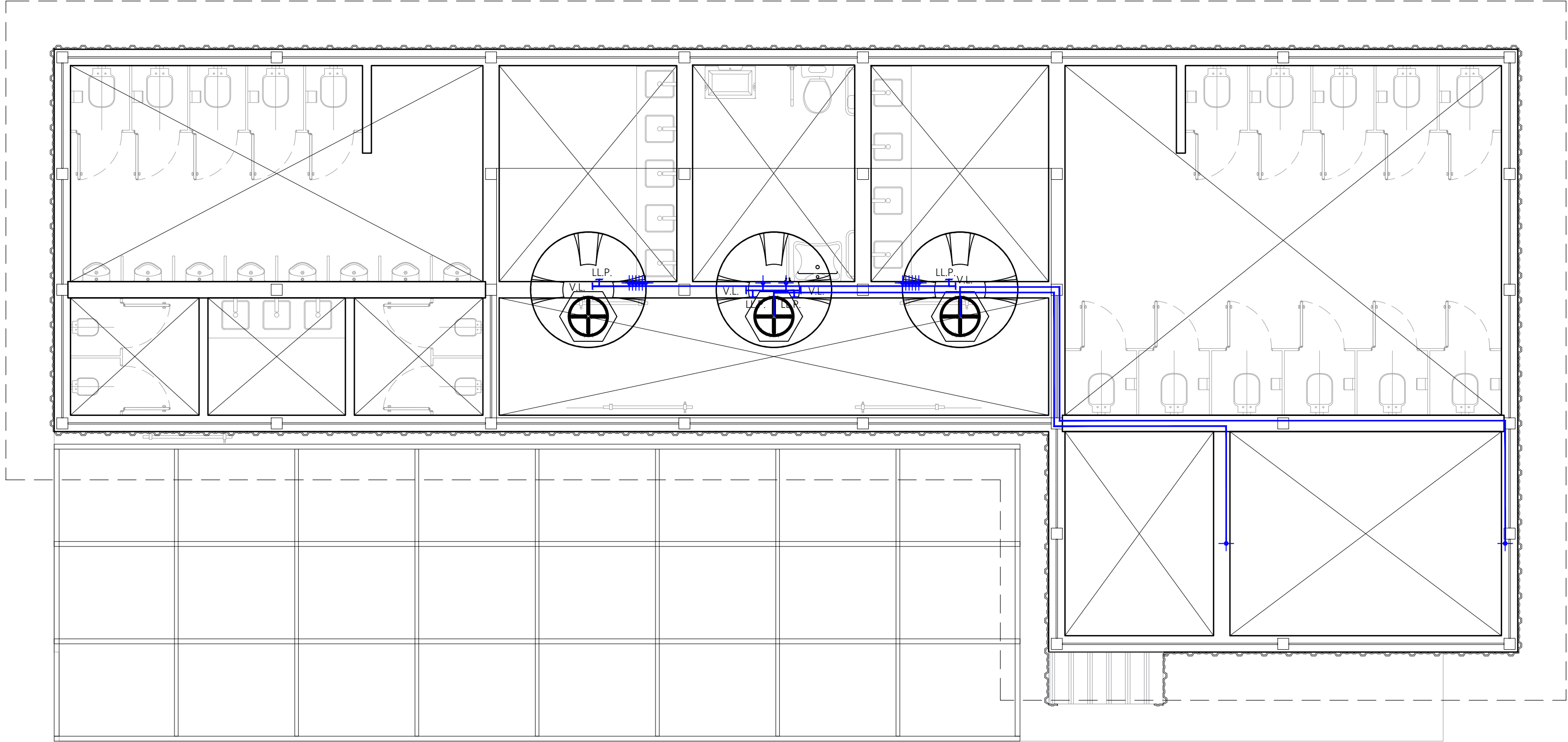
INSTALACIÓN SANITARIA +2,70 ESC 1:50
