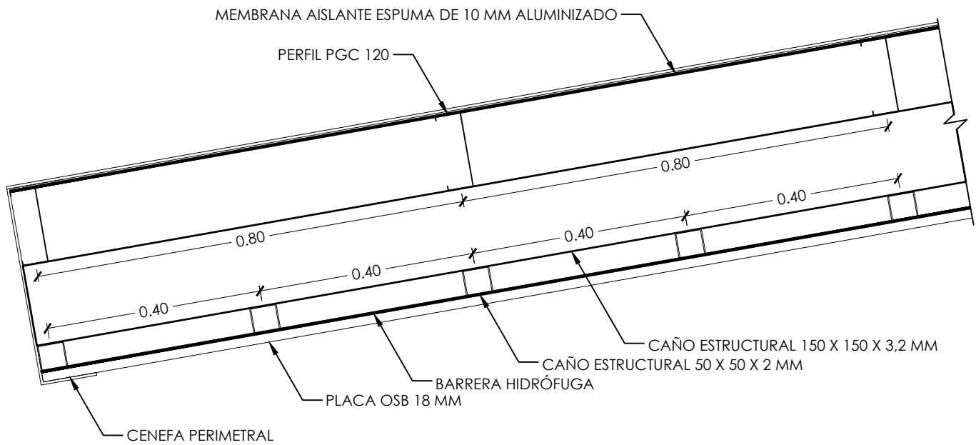
DETALLE CUBIERTA
