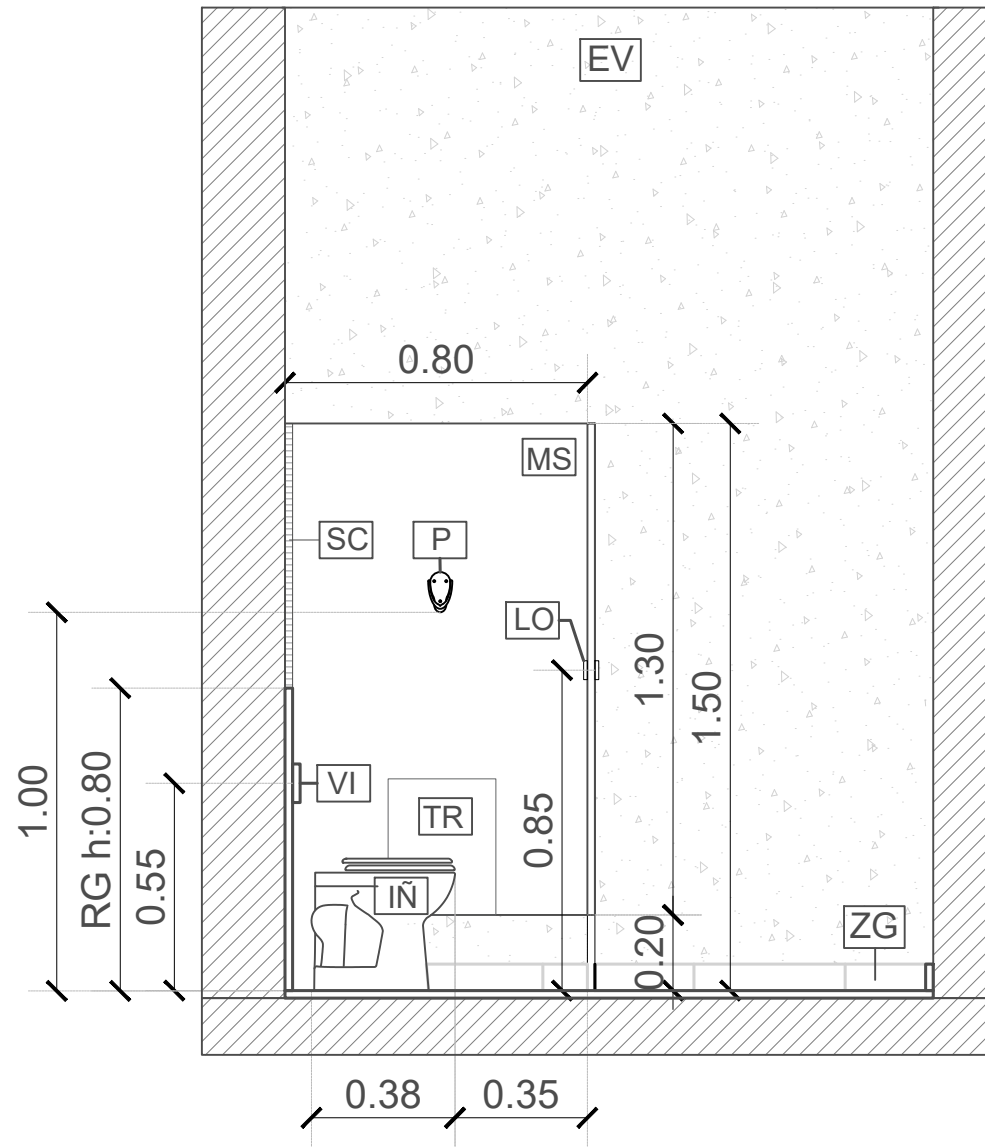
CORTE INODOROS BAÑO FAMILIAR ESC 1:50
