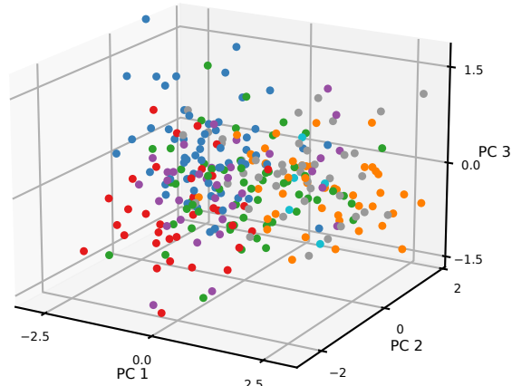
Picture decoder (n=389) NUE031 · cross-task r=0.47^*
