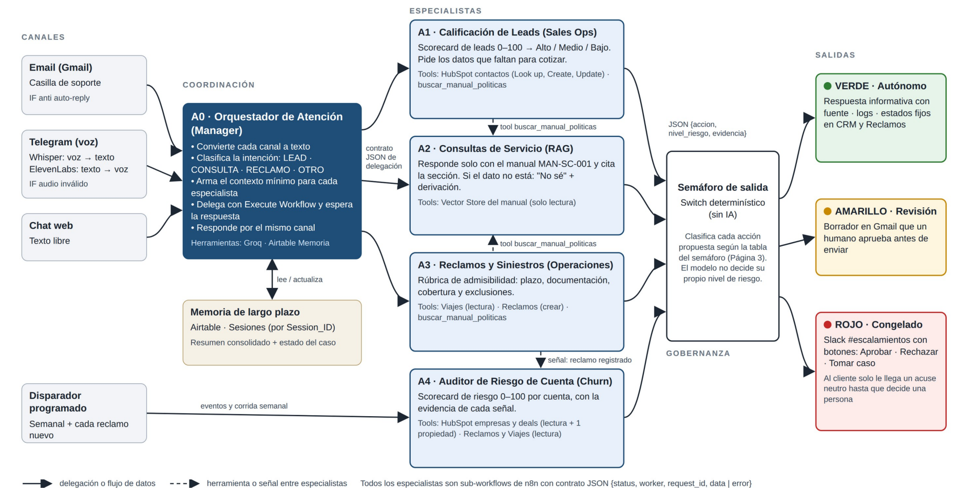
Figura 1. Red de agentes: tres canales de entrada, un orquestador con memoria, cuatro especialistas encapsulados como sub-workflows y un semáforo determinístico que decide qué salidas son autónomas y cuáles quedan congeladas para un humano.
