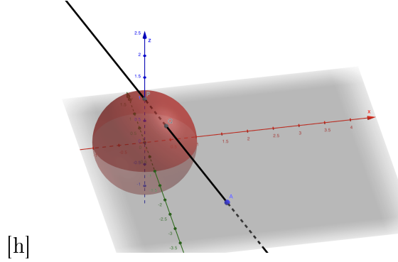
Figura 18.2: Proiezione stereografica e compatificazione di Alexandroff.
