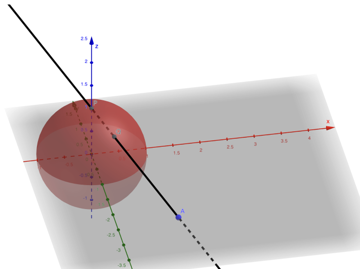
(Proiezione stereografica di S^2 \setminus \{p\} in \mathbb{R}^3 )
