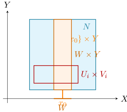
Figura 18.1: Illustrazione del tubo W \times Y \subset N \subset X \times Y DISEGNO DA RIFARE.
