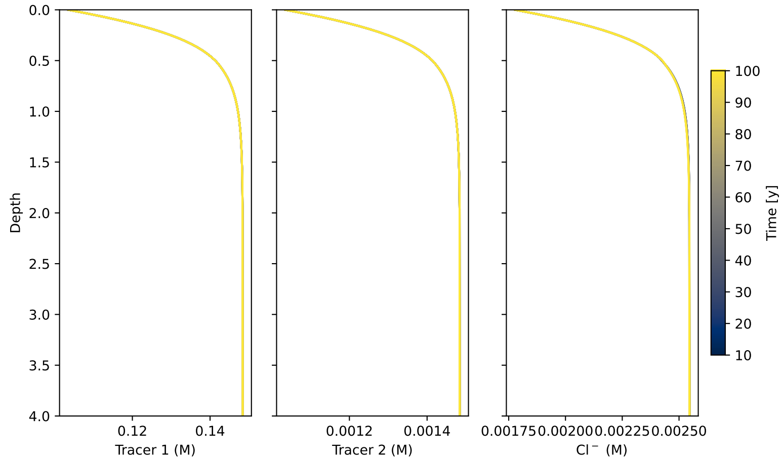
Yolo: Tracer profiles
