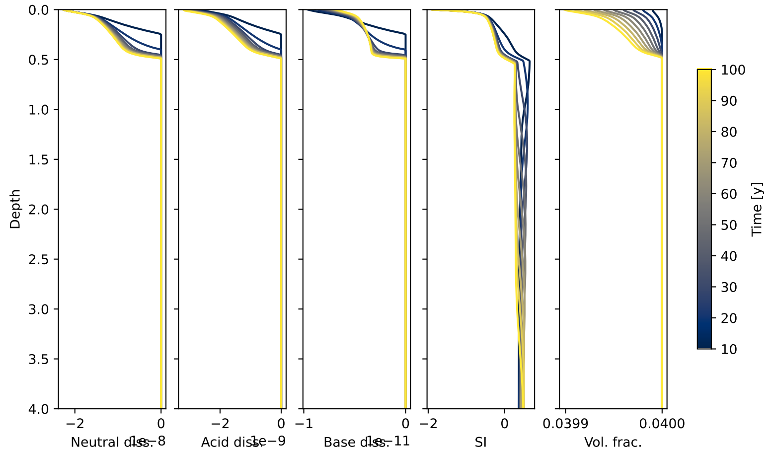
Yolo: K-feldspar dissolution
