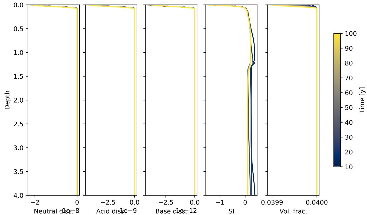
Cecil: K-feldspar dissolution
