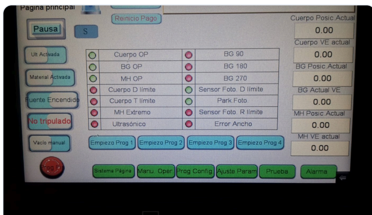
HMI Weinview en español, página principal: estado de sensores (cuerpo, brazo "BG", secador "MH", fotocélulas, ultrasónico), posición y velocidad en vivo, arranque de los 4 programas, modo "No tripulado".
