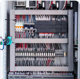
Gabinete de control con PLC y variador.
