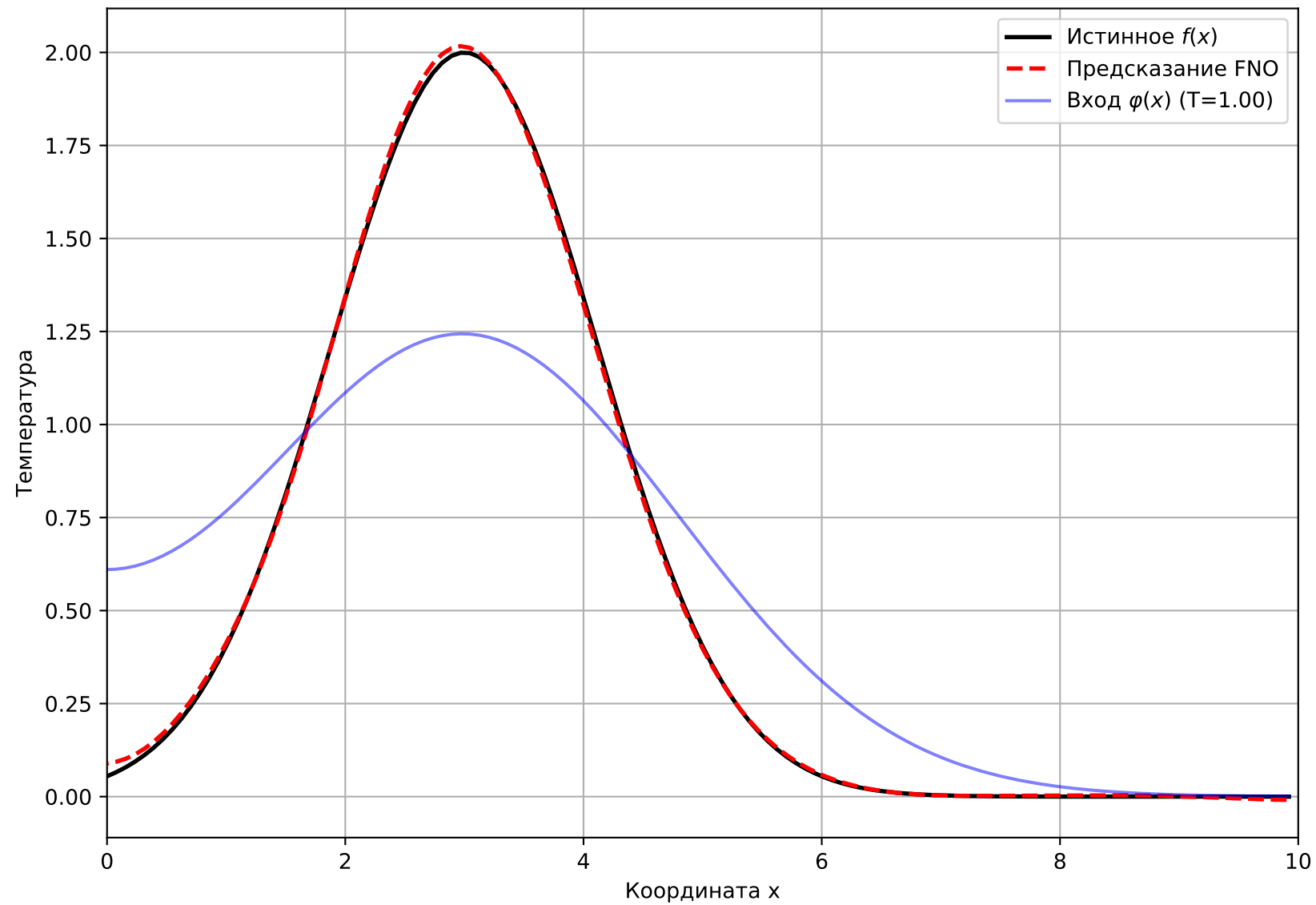
Восстановление f(x) ( T = 1.00 )
