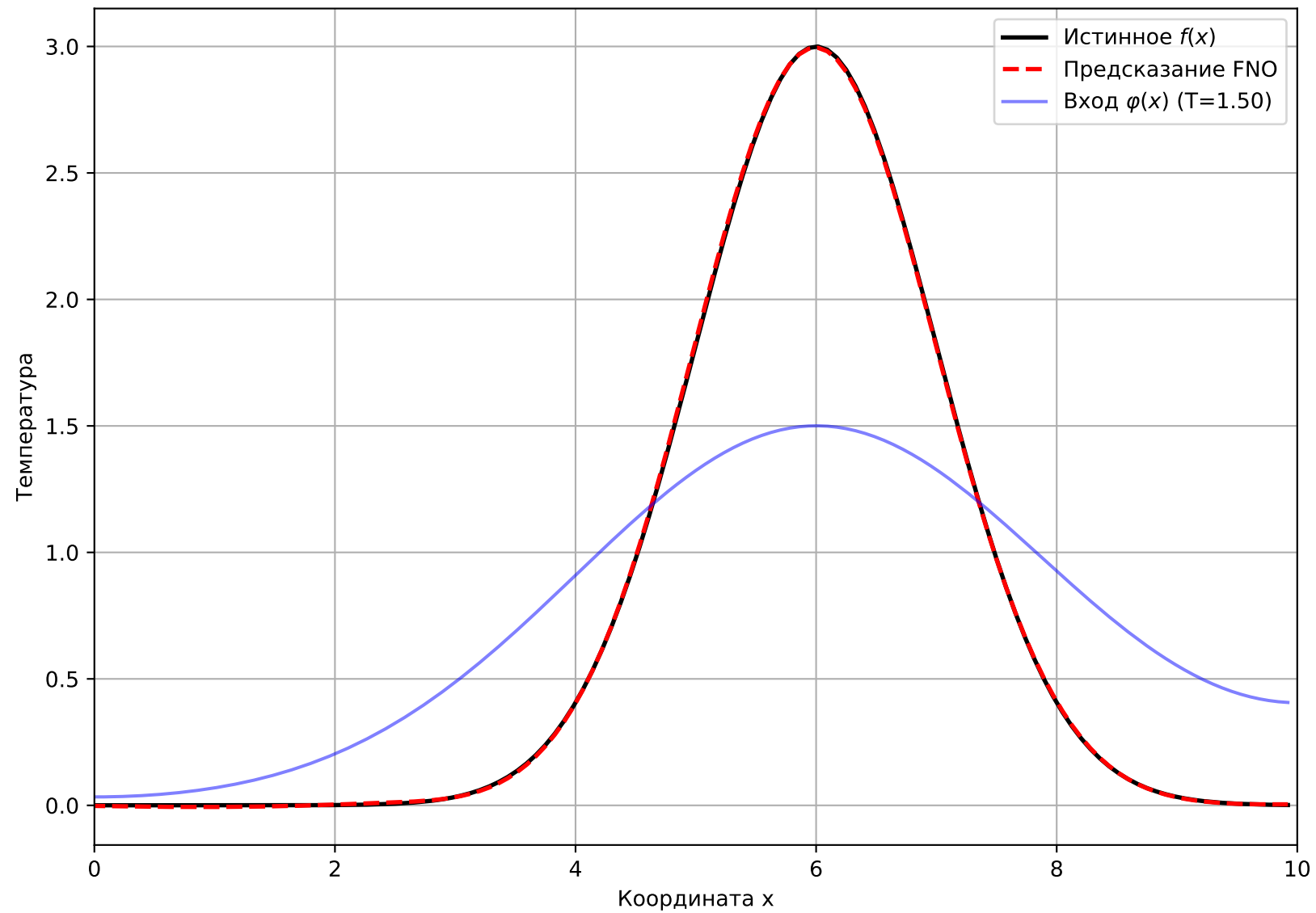
Восстановление f(x) ( T = 1.50 )
