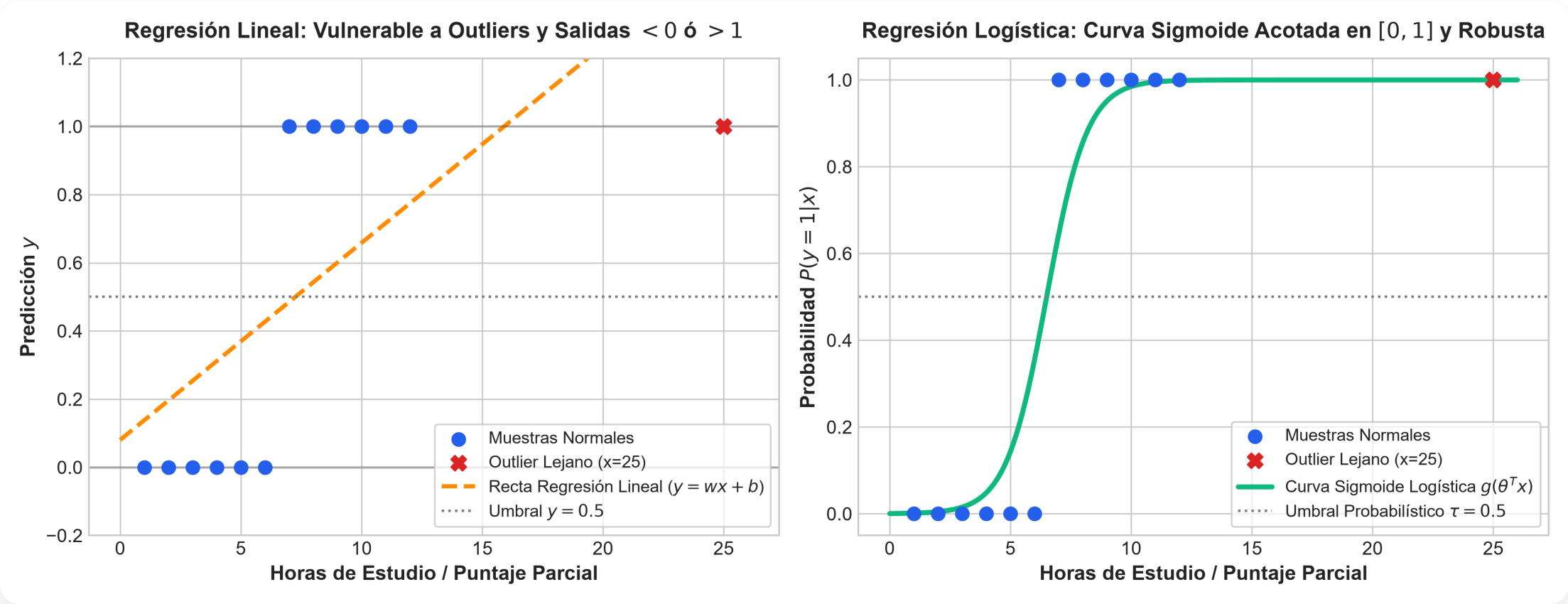
Comparativa: Vulnerabilidad de la Regresión Lineal ante Outliers Izquierda vs. Curva Sigmoide Logística Acotada [0, 1] Derecha
