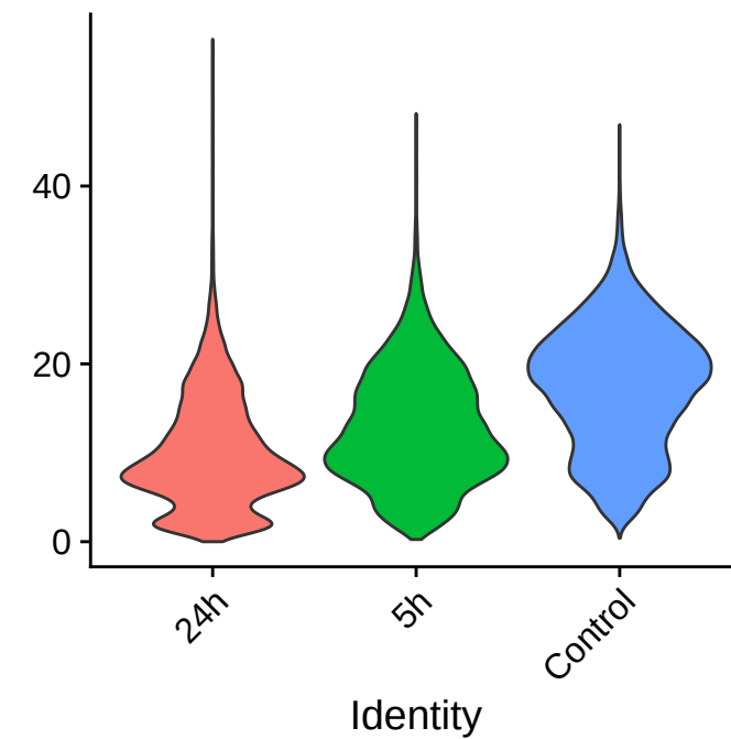
pRibo
