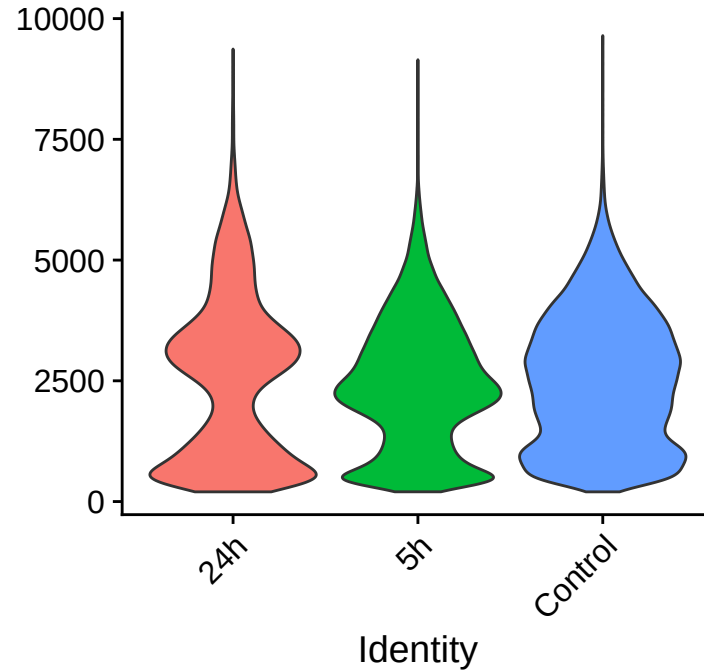
nGene
