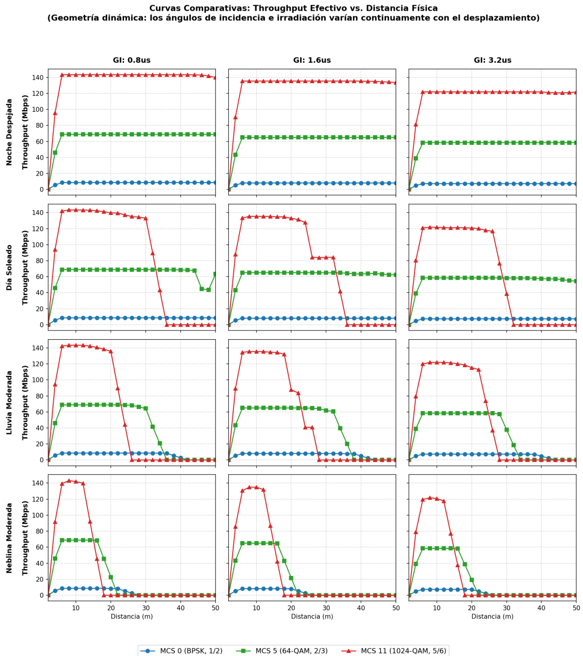
Figura 3.5. Throughput Efectivo (Mbps) vs. Distancia Horizontal (m) en entorno vehicular V2I con barrido hasta 50 metros.
