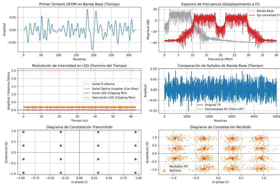
Figura 2.2. Procesamiento paso a paso de las señales y diagramas de constelación del transceptor en un canal óptico de línea de vista (LOS) ideal a una distancia de 3.0 m, en ausencia de ruido solar de fondo ( E_{\text{sol}} = 0 \text{ W/m}^2 ) y con un ruido térmico mínimo ( \sigma_{\text{thermal}}^2 = 10^{-15} \text{ A}^2 ). Se observa la constelación 16-QAM recibida perfectamente ecualizada, logrando una tasa de error de bit de BER = 0.0.
