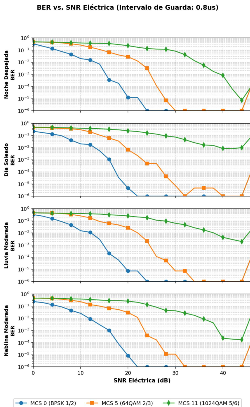
Figura 3.4. Tasa de Error de Bit (BER) vs. SNR Eléctrica (dB) para un Intervalo de Guarda (GI) de 0,8 \mu s (1 columna de 4 filas de escenarios ambientales).
