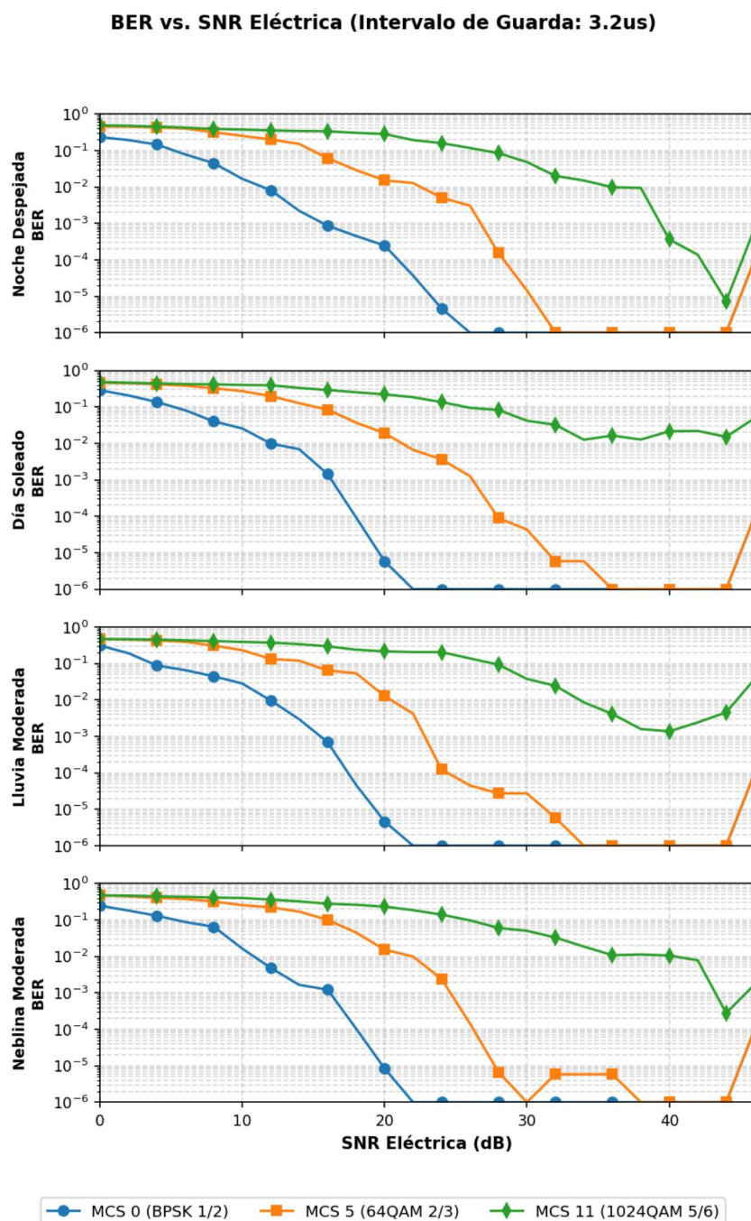
Figura 3.6. Tasa de Error de Bit (BER) vs. SNR Eléctrica (dB) para un Intervalo de Guarda (GI) de 3,2 \mu s (1 columna de 4 filas de escenarios ambientales).
