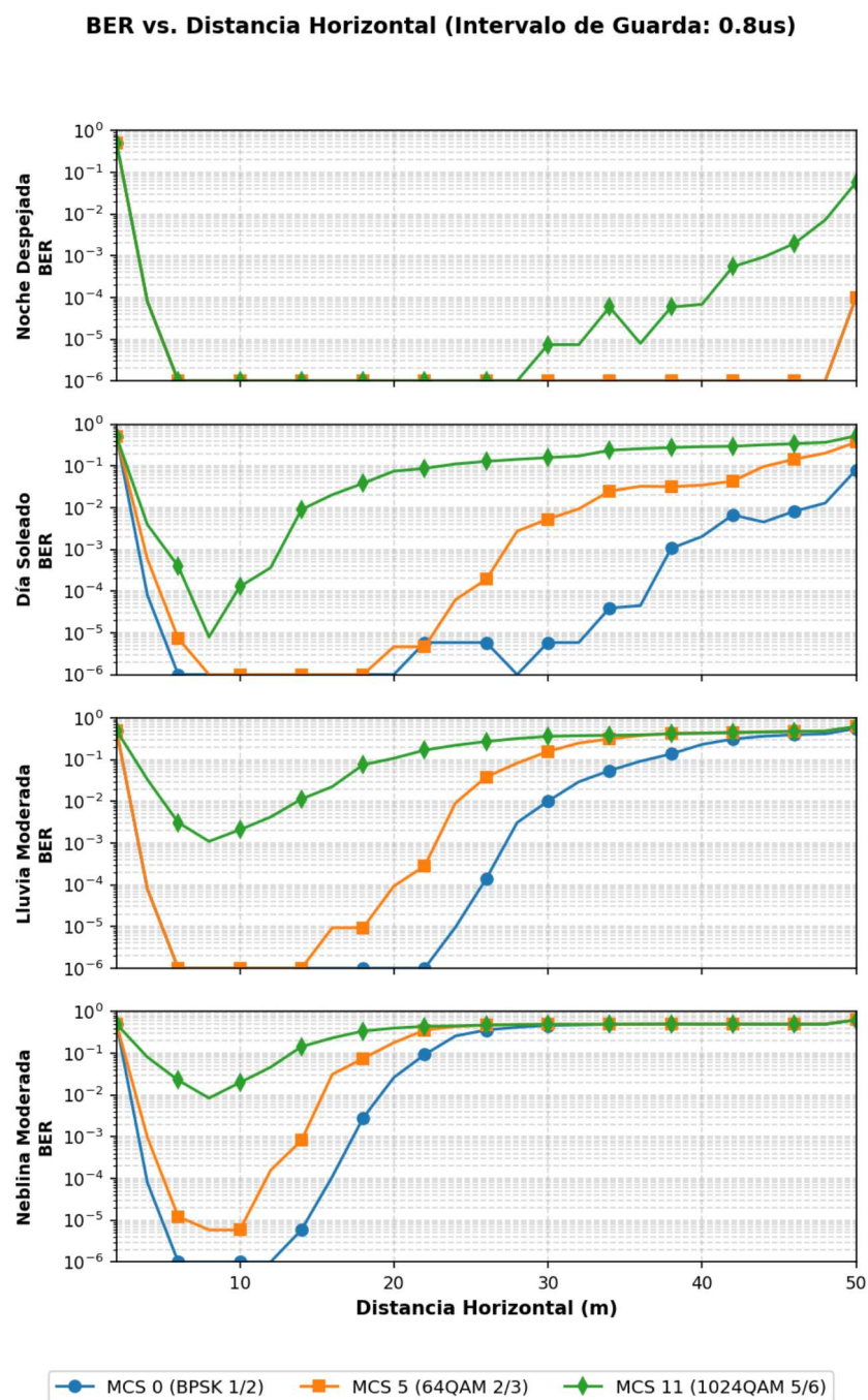
Figura 3.7. Tasa de Error de Bit (BER) vs. Distancia Horizontal (m) para un Intervalo de Guarda (GI) de 0,8 \mu s (1 columna de 4 filas de escenarios ambientales).
