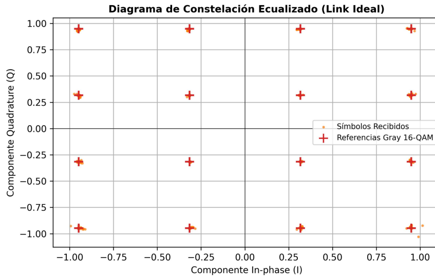
Figura 2.5. Diagrama de constelación ecualizado en el receptor para un esquema 16-QAM bajo un canal óptico ideal libre de interferencias.
