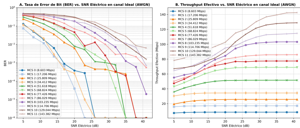
Figura 3.2. Curvas de BER vs. SNR eléctrica teórica en canal AWGN ideal para todos los doce esquemas MCS (del MCS 0 al MCS 11) definidos en el estándar IEEE 802.11bb.
