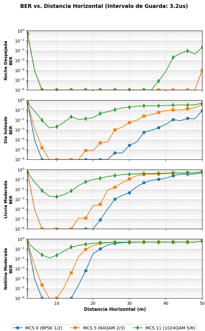
Figura 3.9. Tasa de Error de Bit (BER) vs. Distancia Horizontal (m) para un Intervalo de Guarda (GI) de 3,2 \mu s (1 columna de 4 filas de escenarios ambientales).
