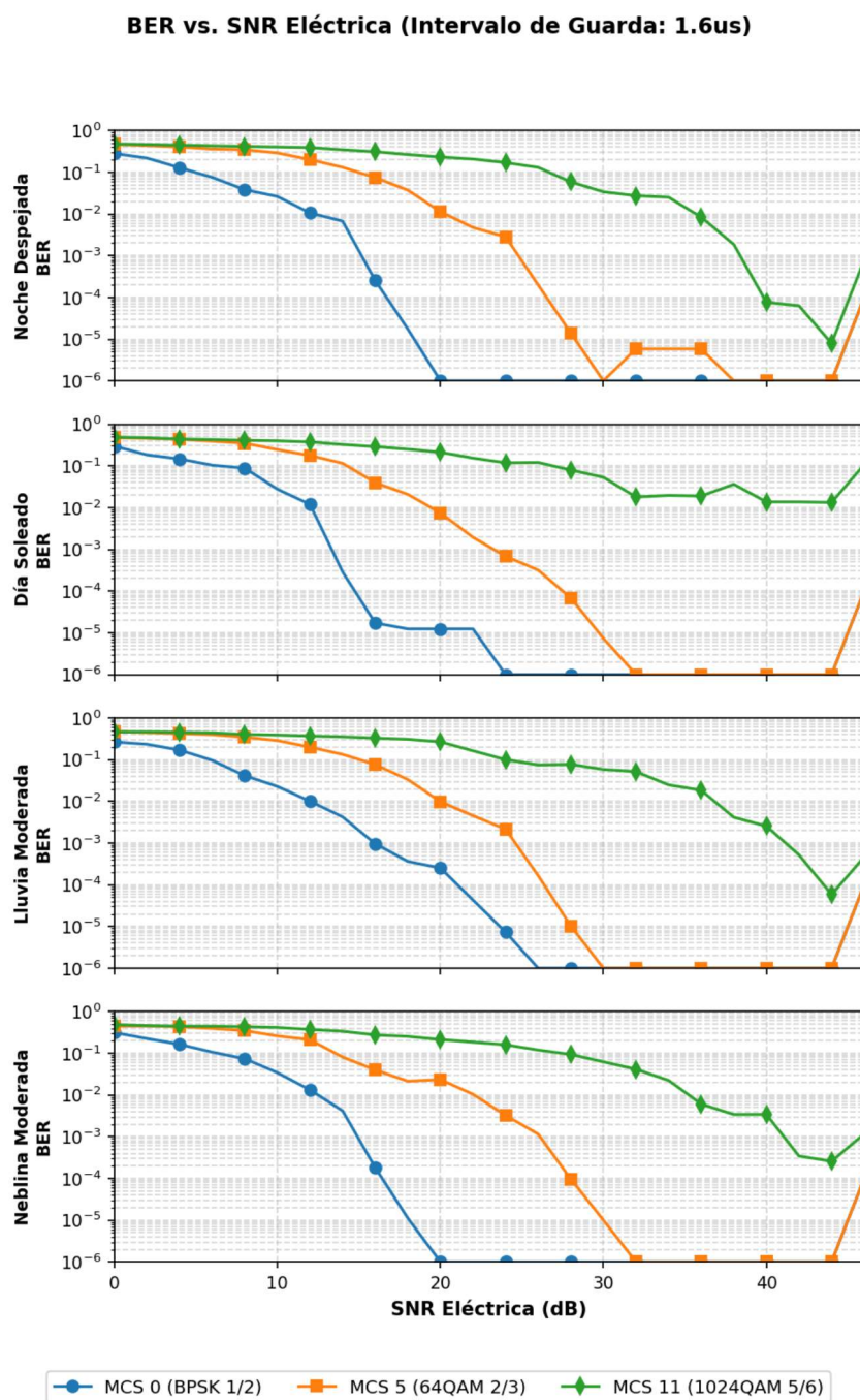
Figura 3.5. Tasa de Error de Bit (BER) vs. SNR Eléctrica (dB) para un Intervalo de Guarda (GI) de 1,6 \mu s (1 columna de 4 filas de escenarios ambientales).
