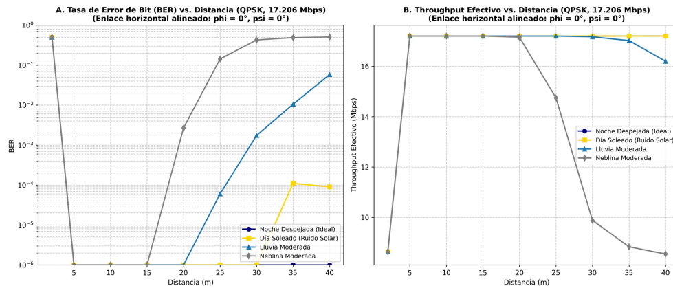
Figura 3.3. Tasa de Error de Bit (BER) y Throughput efectivo en función de la distancia de propagación en enlace horizontal alineado para los cuatro escenarios climáticos.
