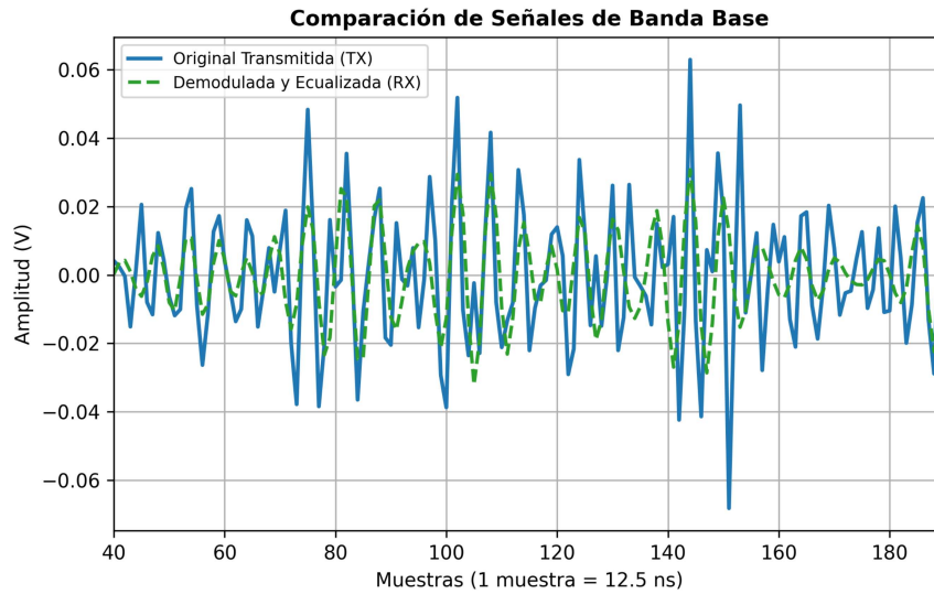
Figura 2.4. Comparación en el dominio del tiempo entre la señal de banda base original transmitida y la señal demodulada y filtrada bajo un enlace ideal sin ruido.
