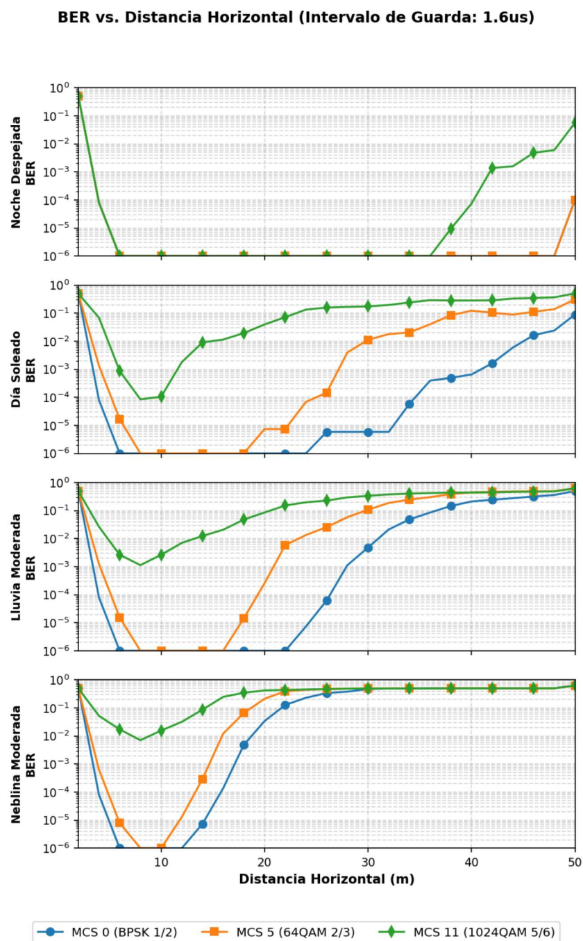
Figura 3.8. Tasa de Error de Bit (BER) vs. Distancia Horizontal (m) para un Intervalo de Guarda (GI) de 1,6 \mu s (1 columna de 4 filas de escenarios ambientales).
