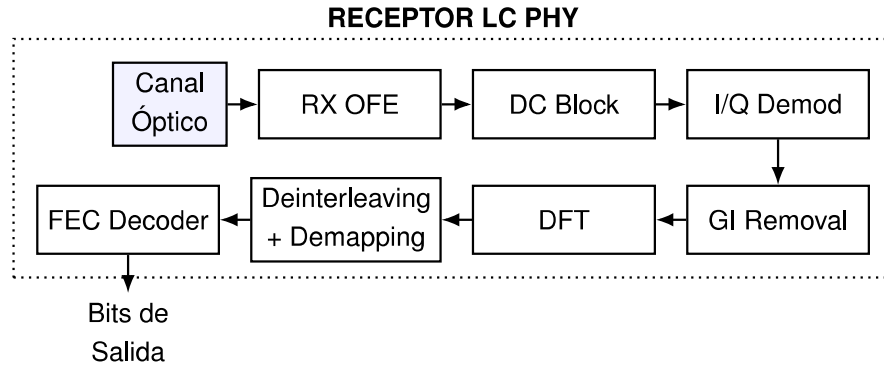
Figura 1.2. Diagrama de bloques funcionales del receptor de la capa física (LC PHY) según el estándar.
