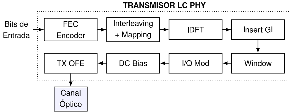
Figura 1.1. Diagrama de bloques funcionales del transmisor de la capa física (LC PHY) según el estándar.
