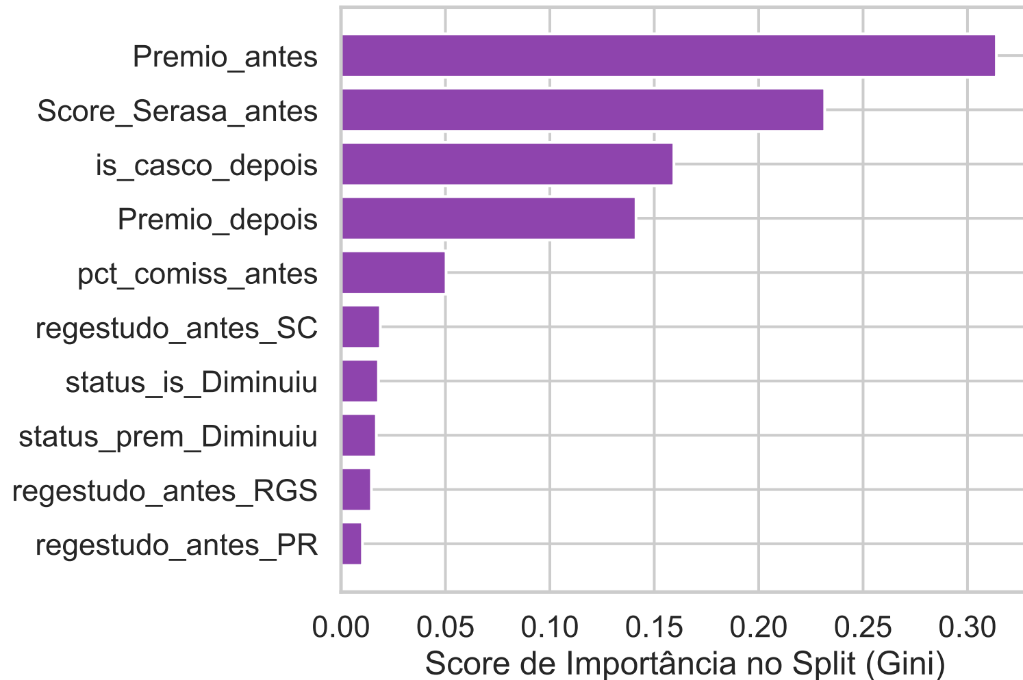
Top 10 Variaveis Importantes (Random Forest)
