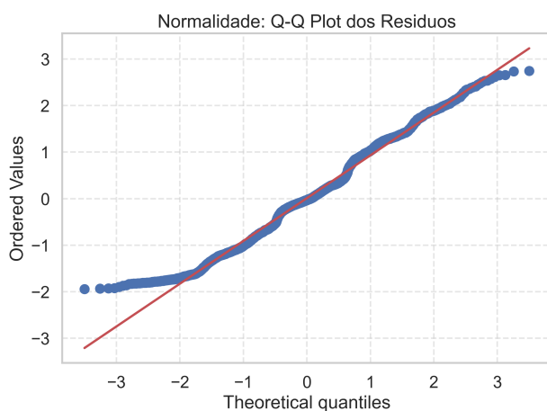
Normalidade: Q-Q Plot
