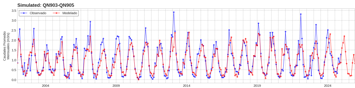
Figure 20: Caudal Incremental Promedio Mensual (m³/s) en QN-903 + QN-904 + QN-905 (2002–2025)
