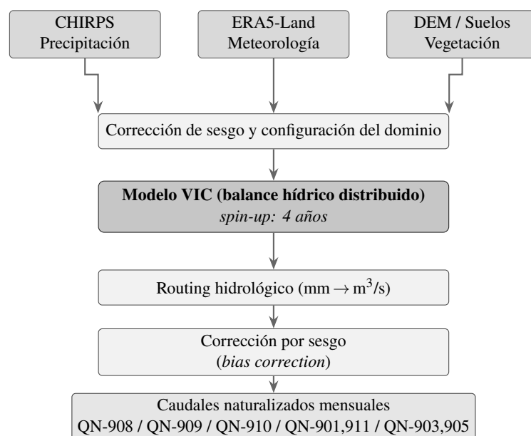
Figure 1: Esquema metodológico para la estimación de caudales promedio mensuales naturales utilizando información satelital, reanálisis climático y corrección por sesgo.
