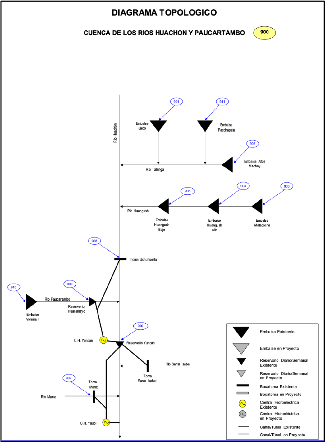
Figure 3: Diagrama Topológico. Cuenca de los Ríos Huachón y Paucartambo
