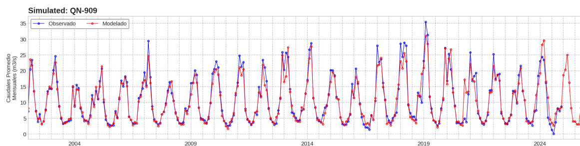
Figure 18: Caudal Incremental Promedio Mensual ( \text{m}^3/\text{s} ) en QN-909 Huallamayo (2002–2025)
