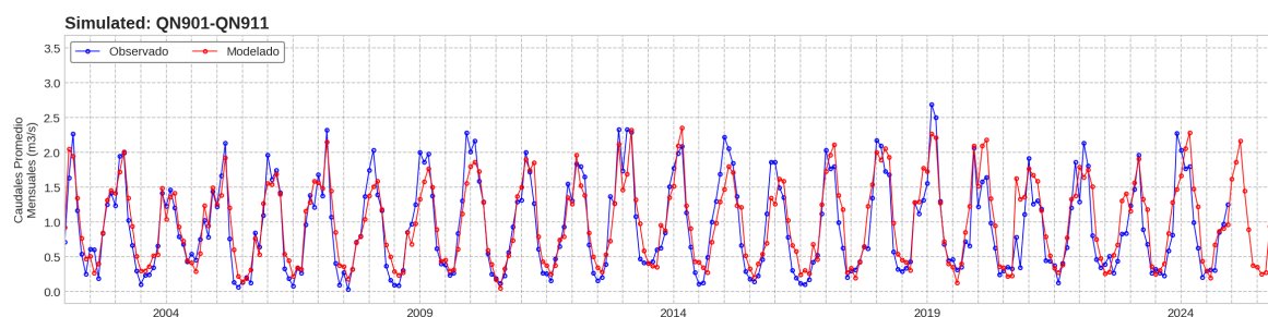
Figure 19: Caudal Incremental Promedio Mensual ( \text{m}^3/\text{s} ) en QN-901 + QN-902 + QN-911 (2002–2025)
