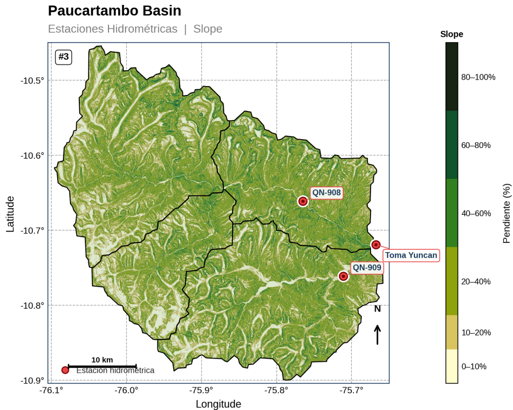
Figure 16: Mapa de Distribución de Pendientes (Fuente: Estudio hidrológico C.H. Yuncán 2025)
