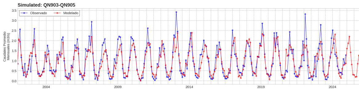
Figure 20: Caudal Incremental Promedio Mensual ( \text{m}^3/\text{s} ) en QN-903 + QN-904 + QN-905 (2002–2025)
