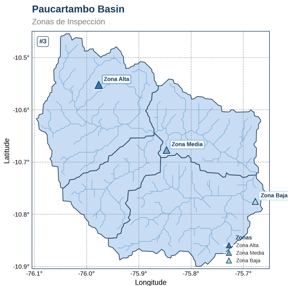
Figure 4: Ubicación de estaciones virtuales para las zonas alta (EstAltaWS), media (EstMediaWS) y baja (EstBajaWS) de la cuenca (Fuente: Estudio hidrológico C.H. Yuncán 2025)
