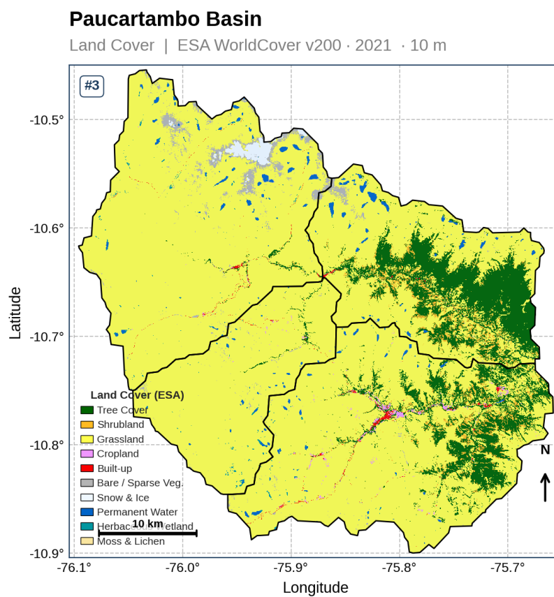
Figure 15: Mapa de Distribución de Cobertura Vegetal (Fuente: Estudio hidrológico C.H. Yuncán 2025)
