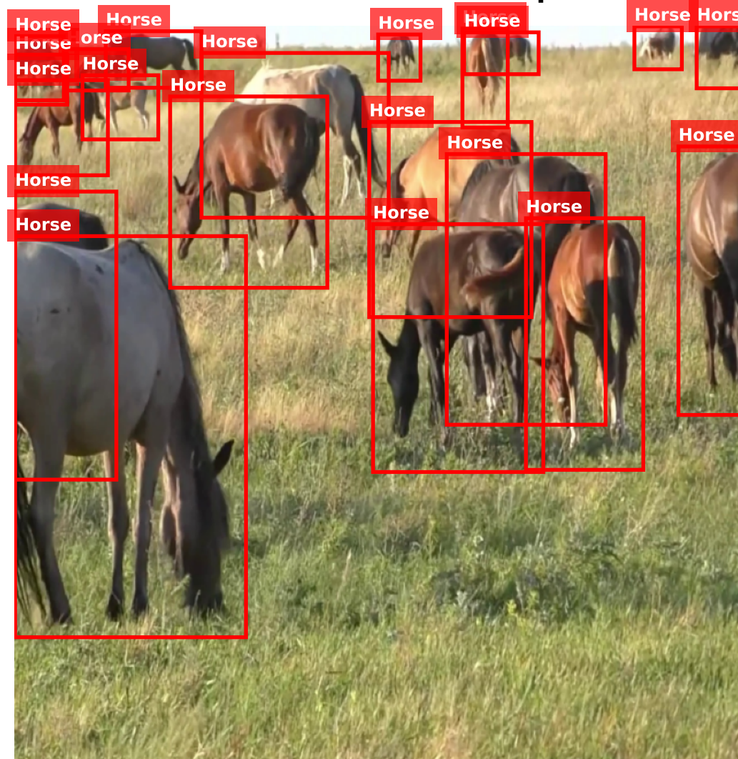
2. RandomResizedCrop
