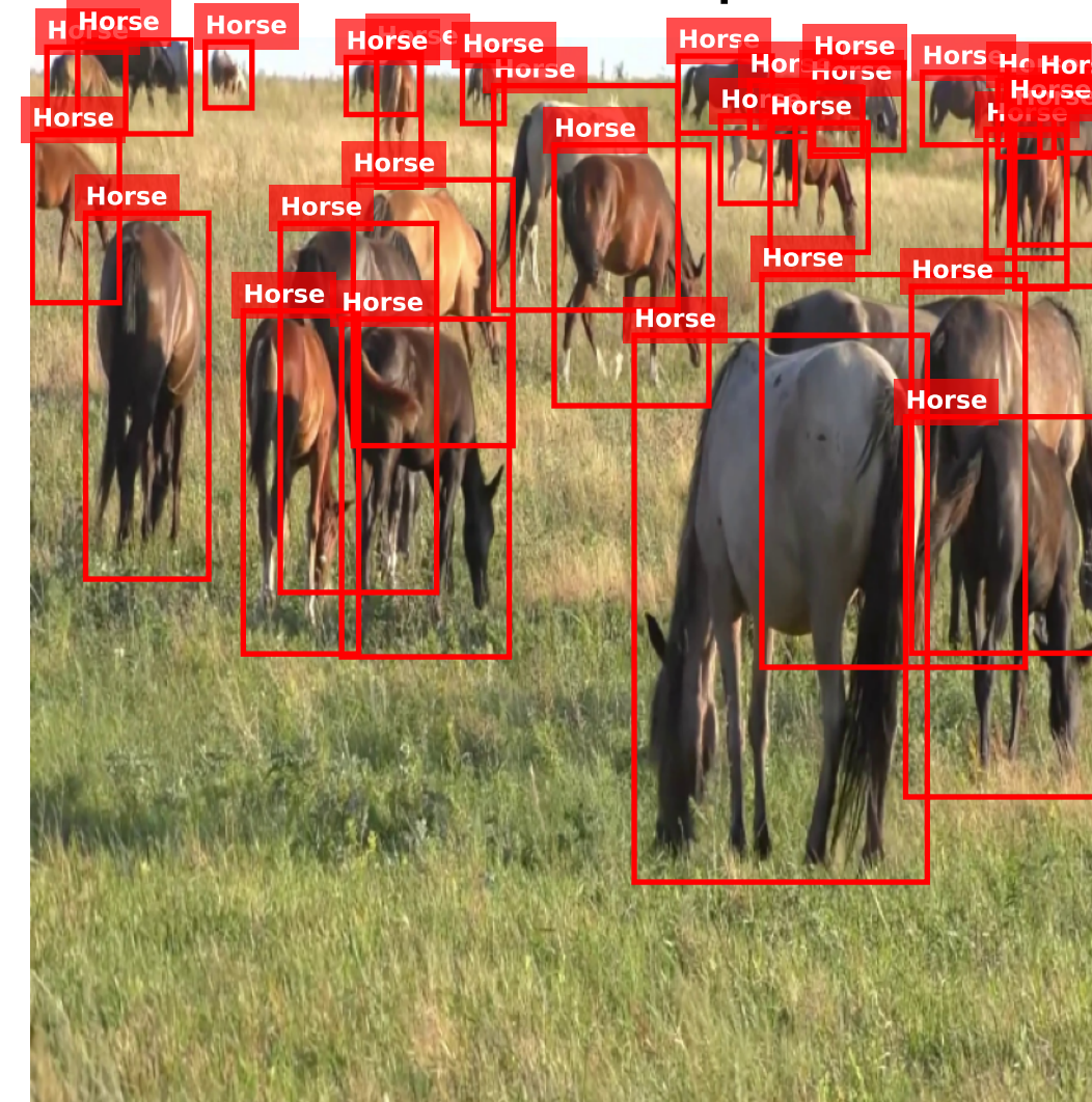
3. HorizontalFlip
