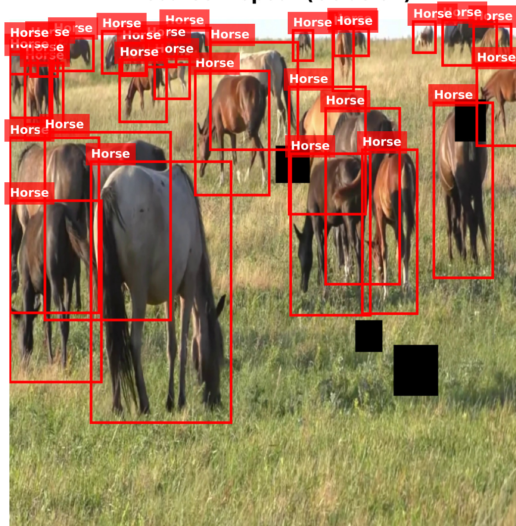
4. CoarseDropout (Oclusión)
