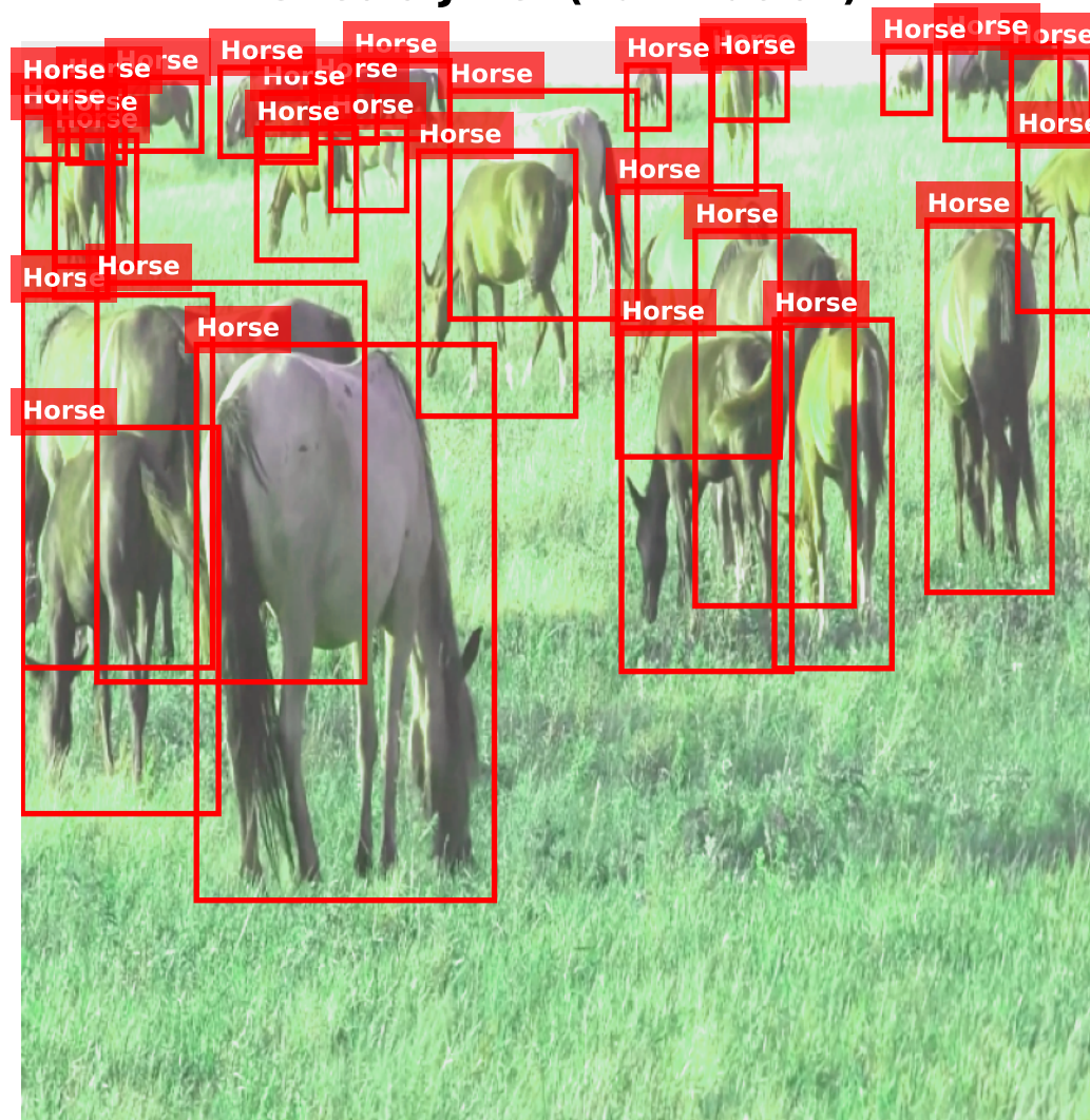
5. ColorJitter (Iluminación)
