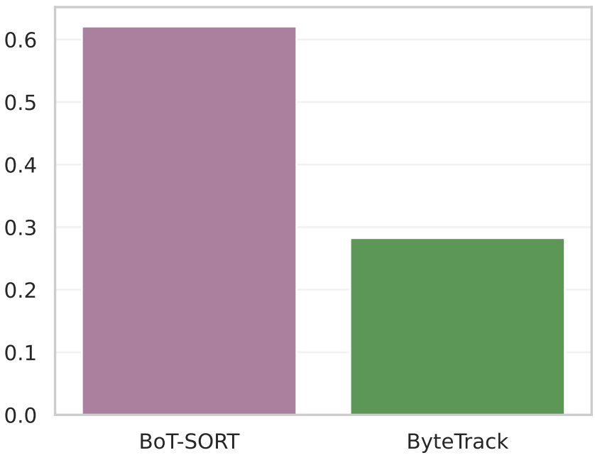
Precision ↑
