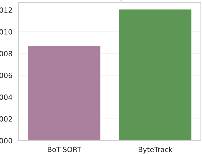
PT/obj
