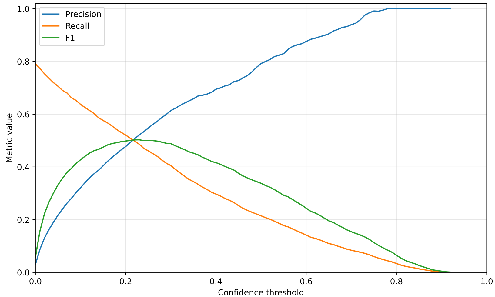
Precision / Recall / F1 vs Confidence Threshold
