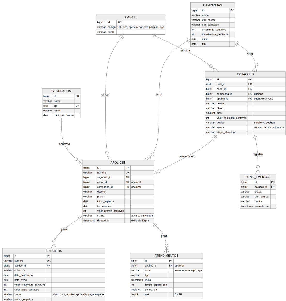
Figura 1: Diagrama de entidade e relacionamento (também em docs/der.svg).
