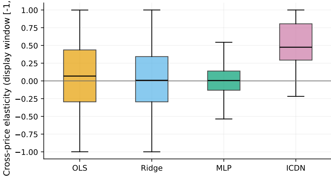
Dominick (beer) — cross-price
