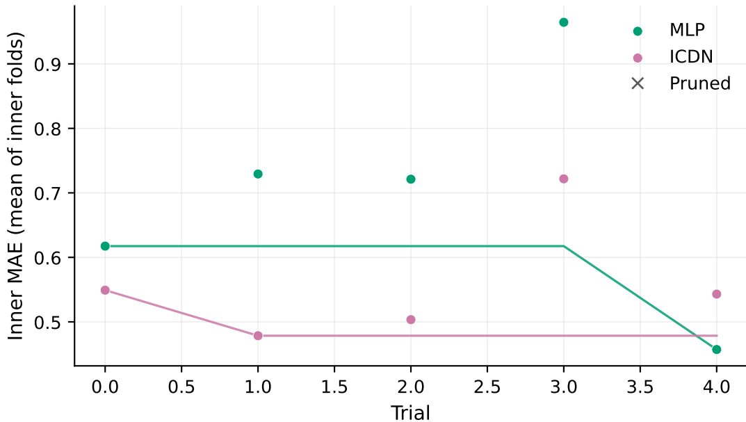
Optuna fold2 — Dominick (beer)
